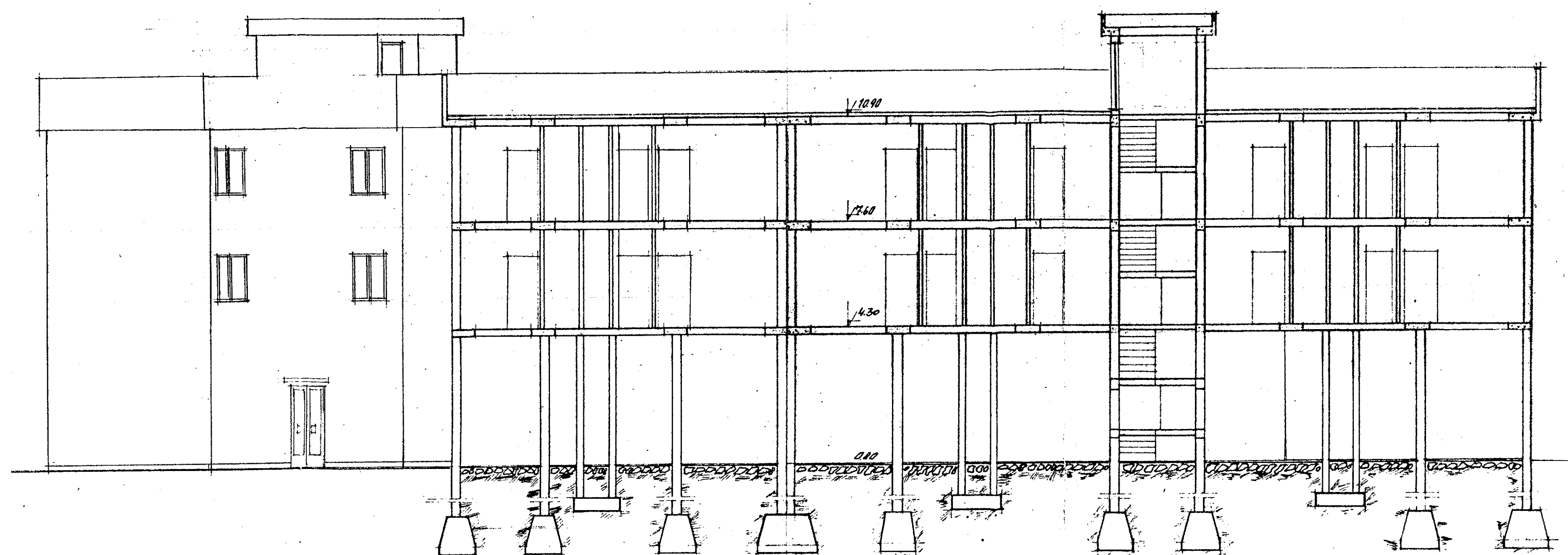
SEZIONE "A - A"
