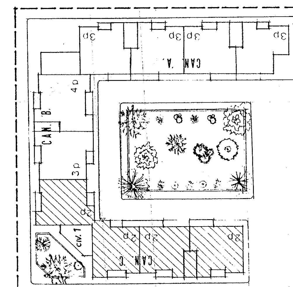
STRALCIO PLANIMETRICO 1:500
