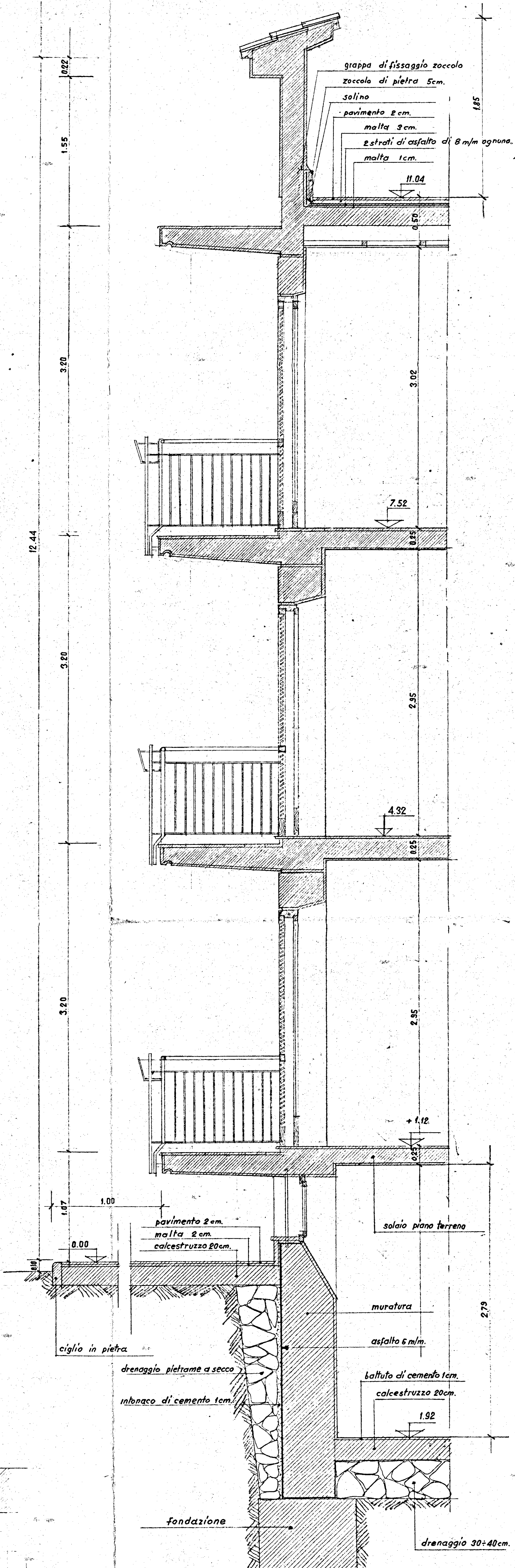
SEZIONE: A-A
