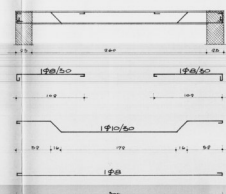
ARMATURA PIANER OTTOLO
