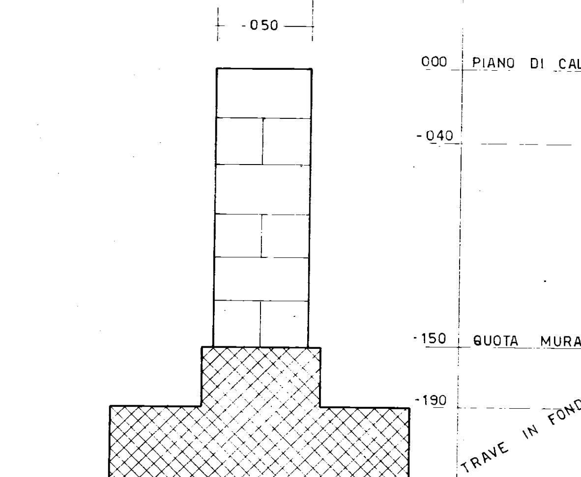
SEZIONE MURATO
