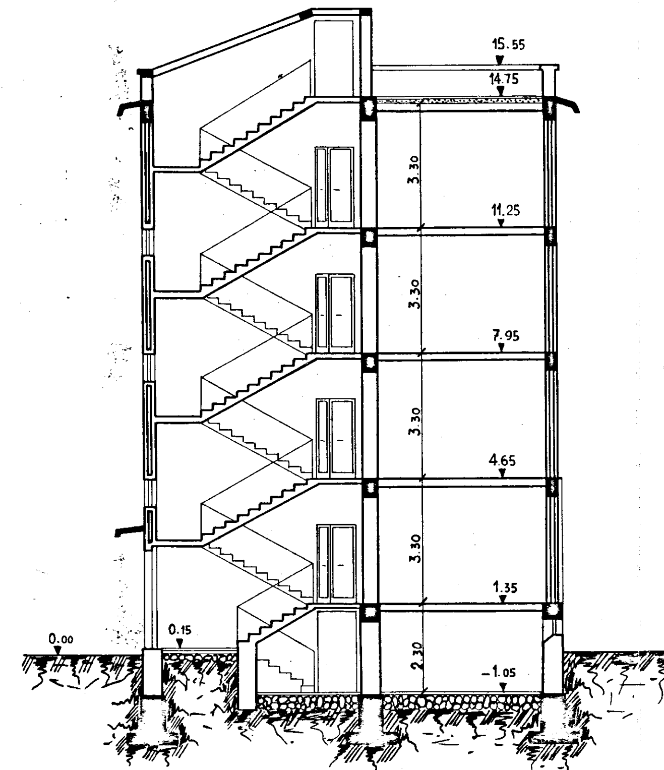
Sezione A.B.
