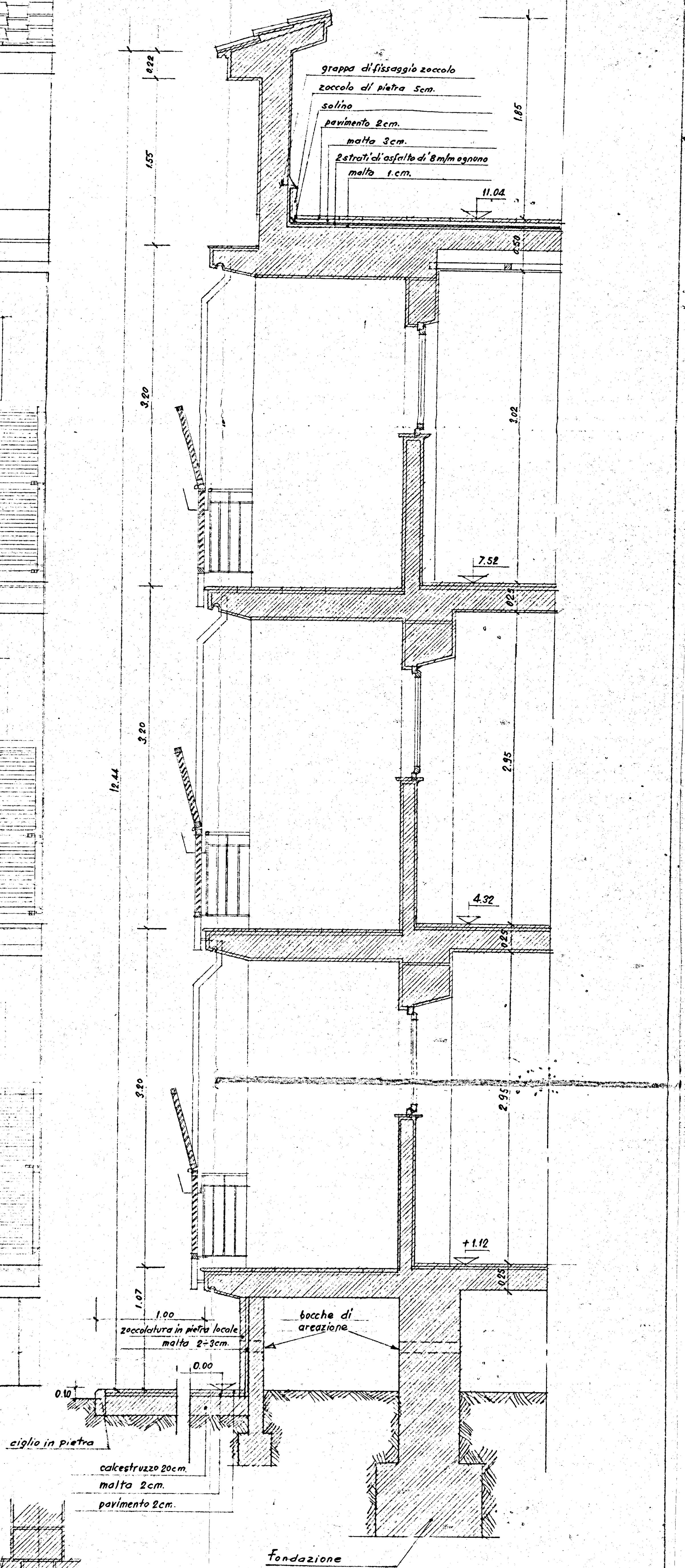
SEZIONE A-A
