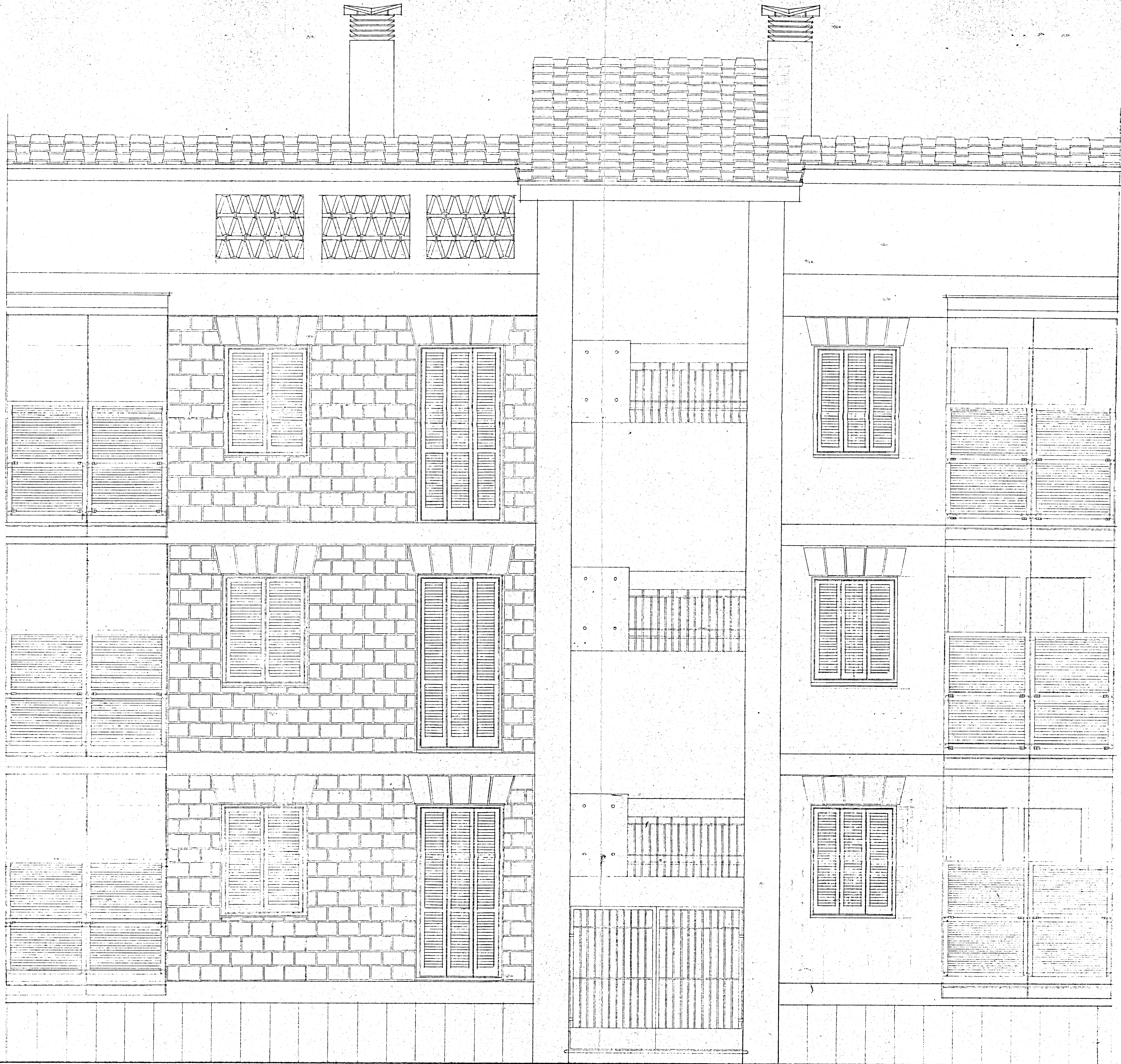
PROSPETTO
