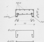
SEZIONE TRAVE DI CODONAMENTO POSTICO RADA 1/20
