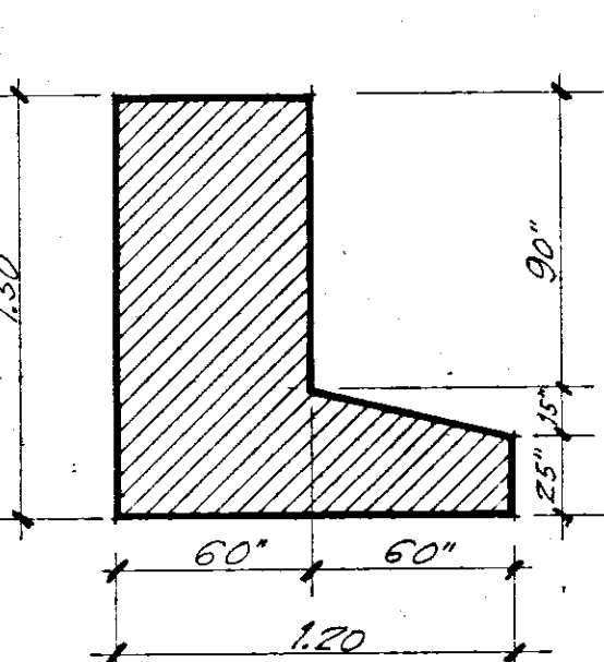
SEZIONE TRAVE DI GIUNTO RAPP. 1:25
