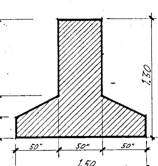
SEZIONE TRAVE TIPO RAPP. 1:25
