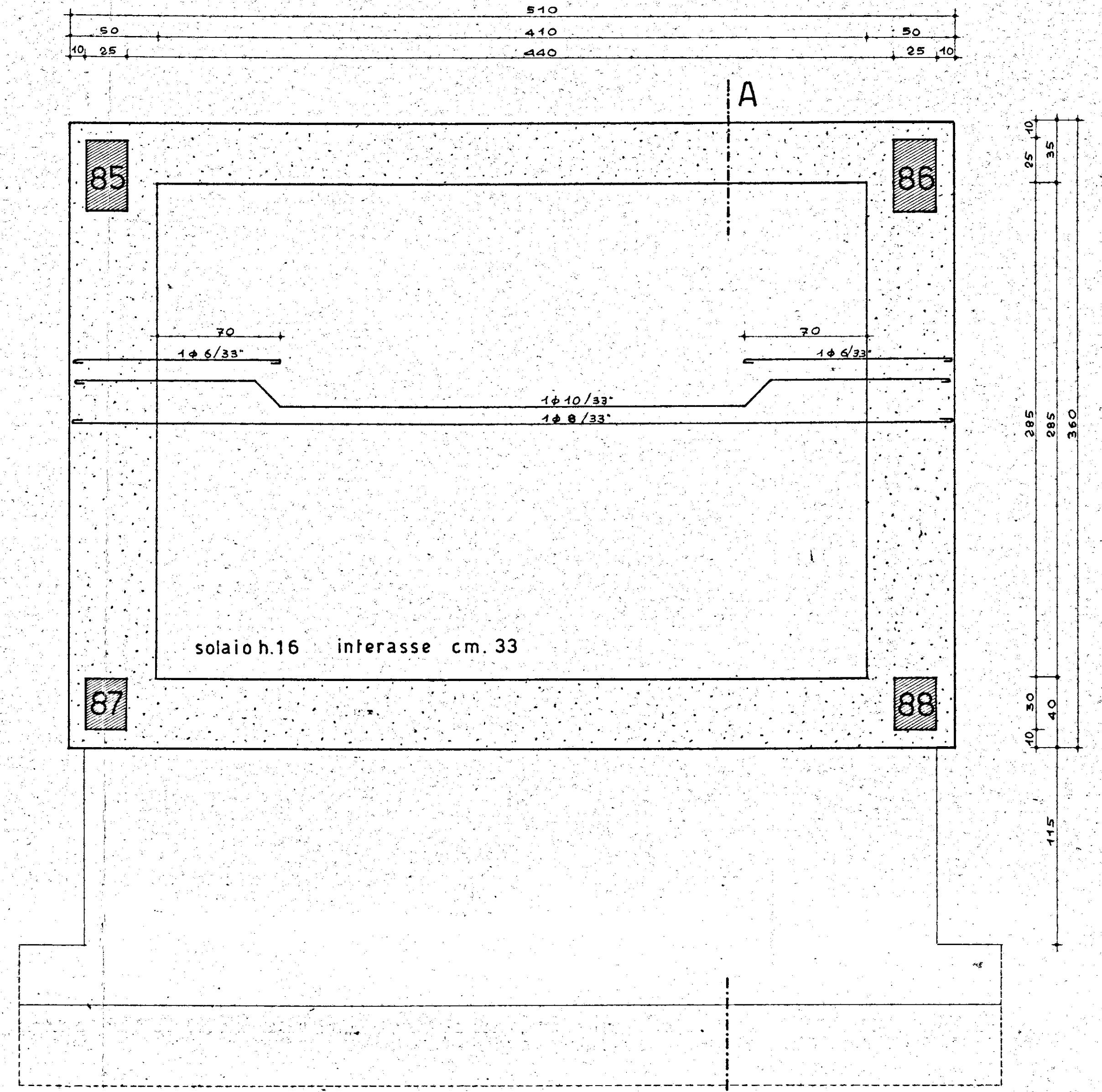
copertura torrino
