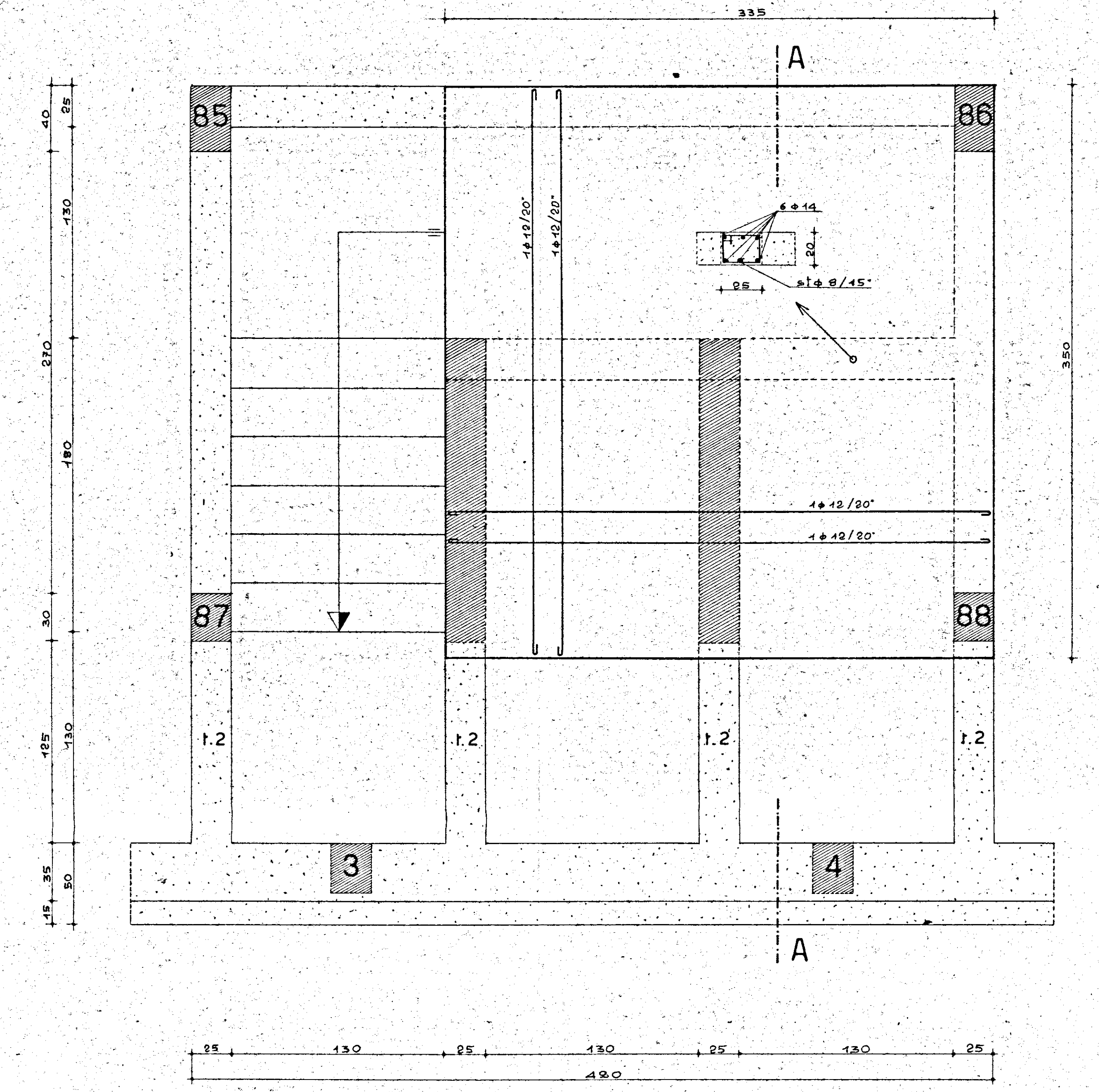
pianta torrino
