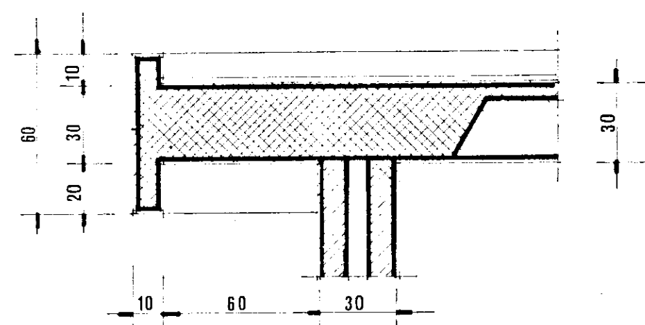
particolare A-A rapp. 1:20
