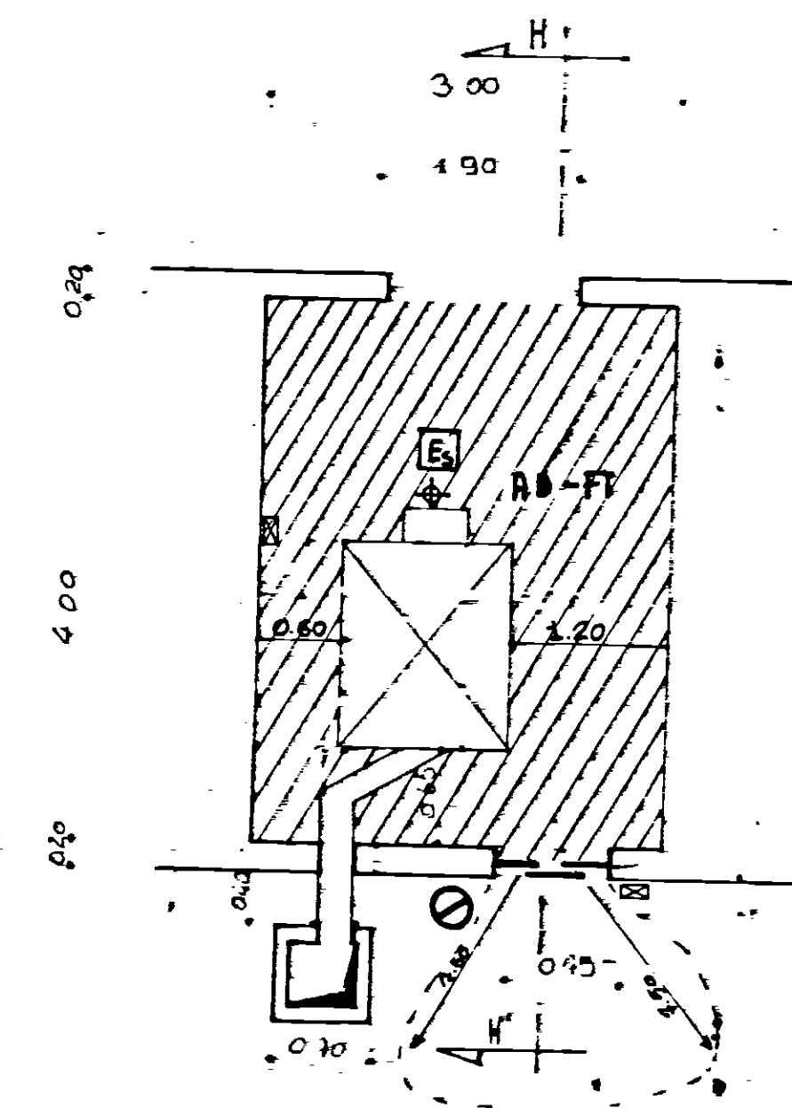
RILIEVO Pianta CENTRALE TERMICA
