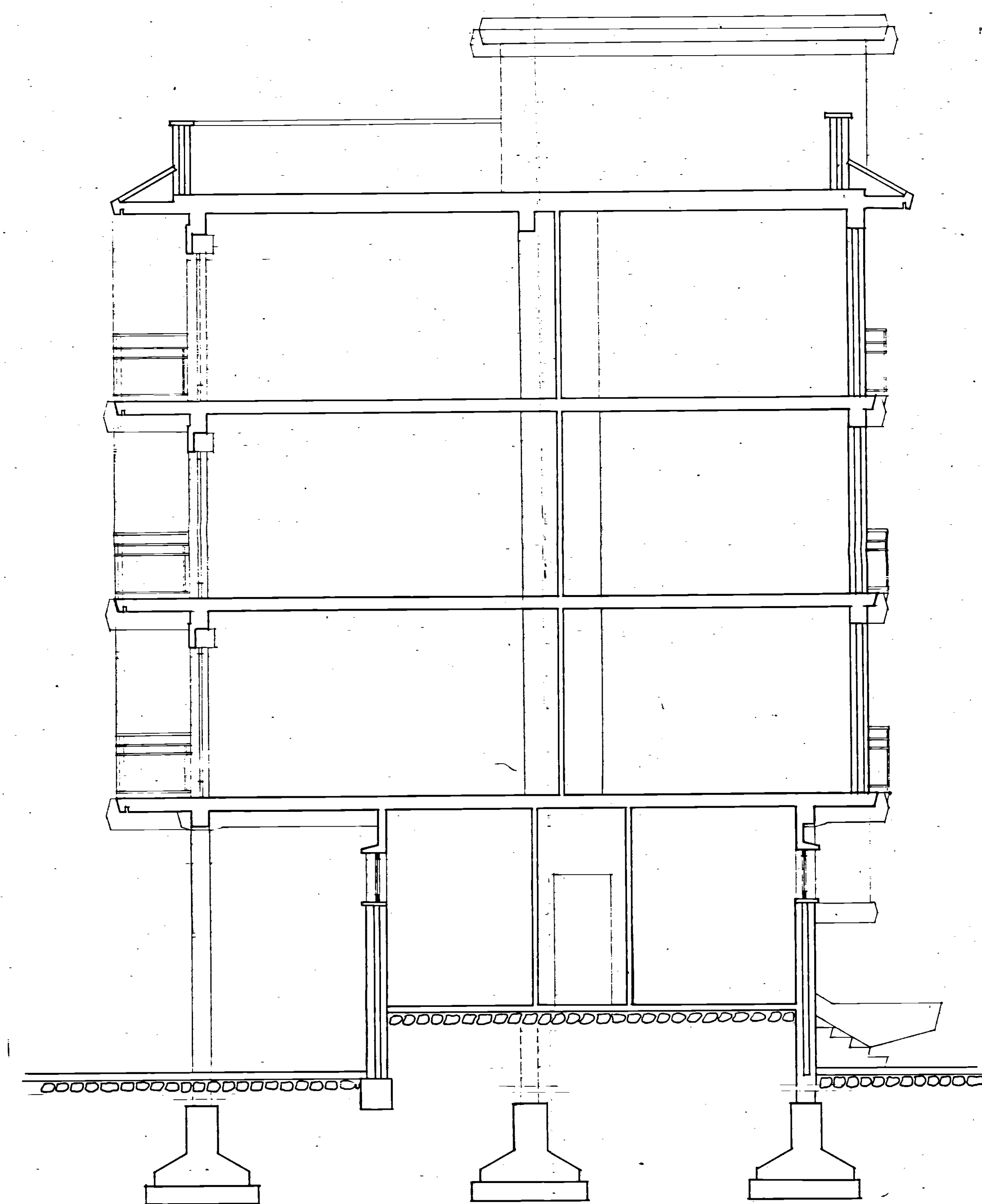
- SEZIONE a-a -
