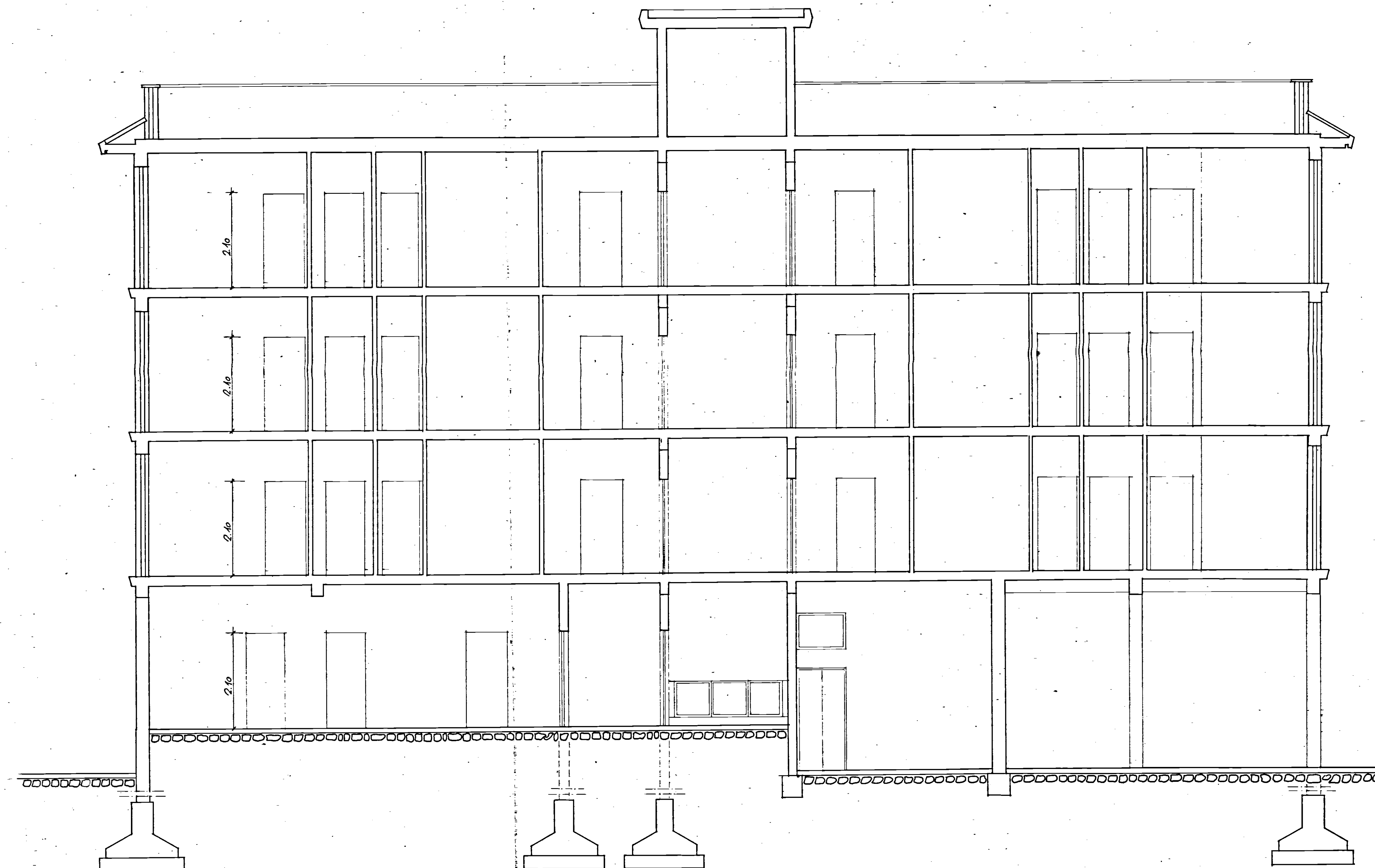
- SEZIONE c-c -
