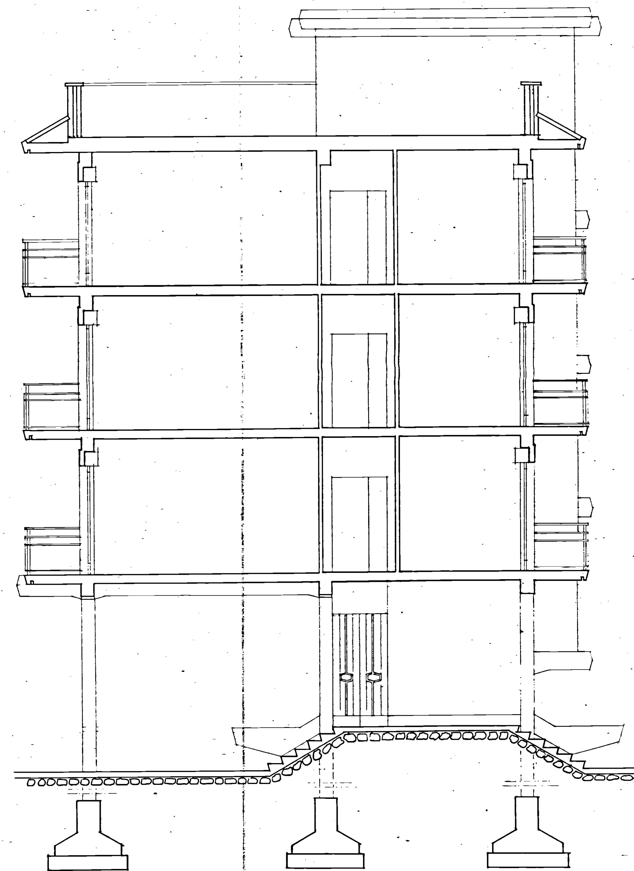
- SEZIONE b-b -
