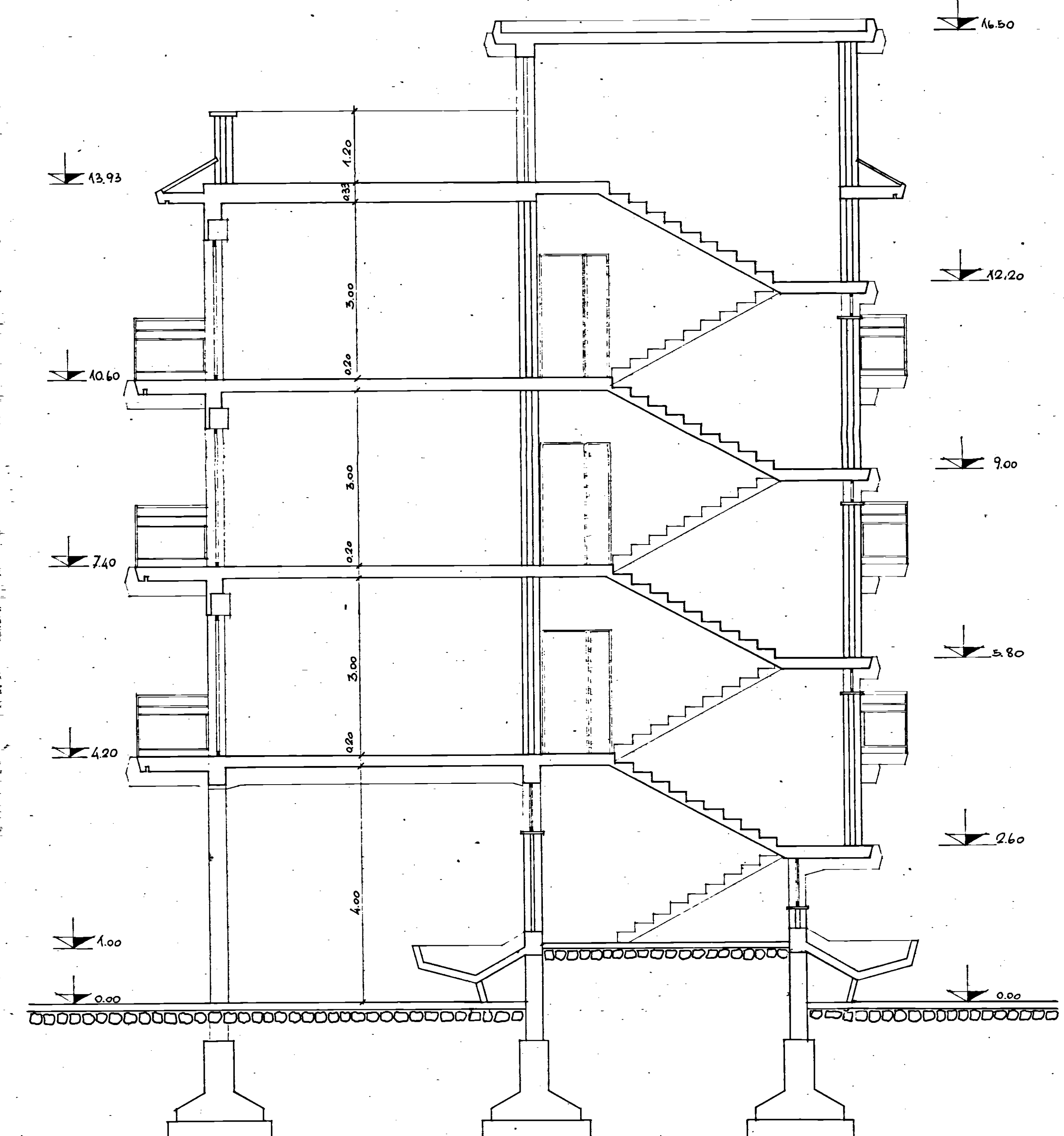
- SEZIONE d-d -
