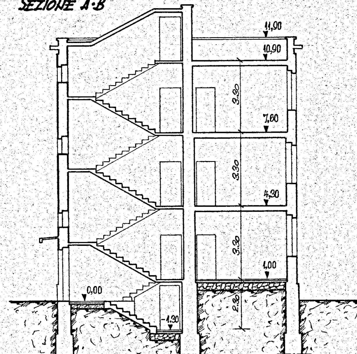
SEZIONE A-B
