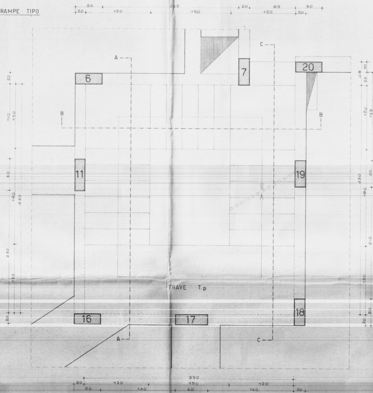
TRAVE T.p
