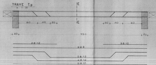
TRAVE T.p
