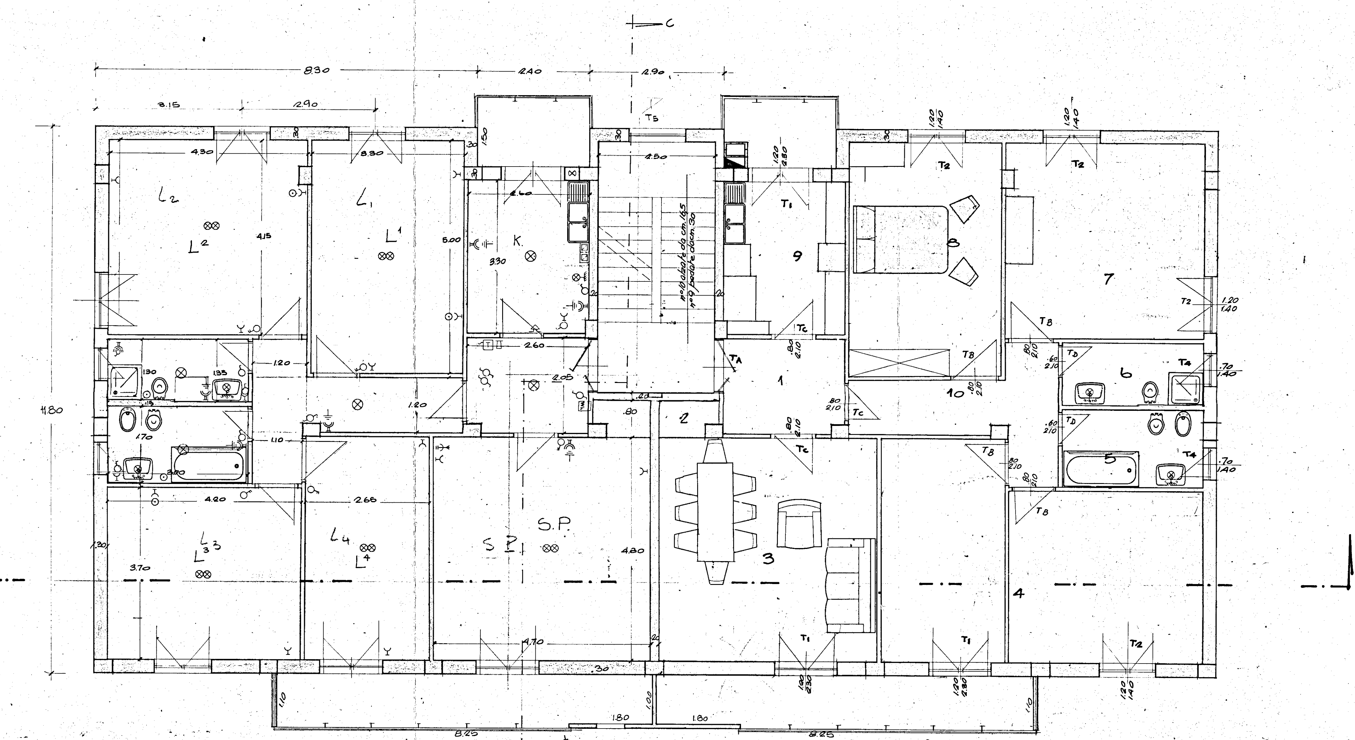
pianta piano tipo
