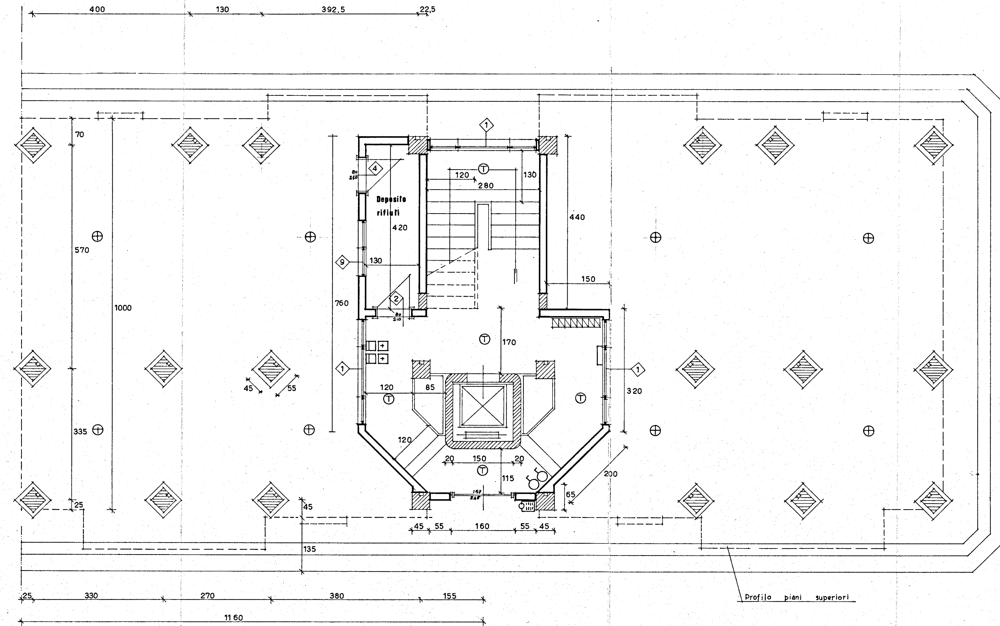
PIANO TERRA (variante per palazzine in linea)
