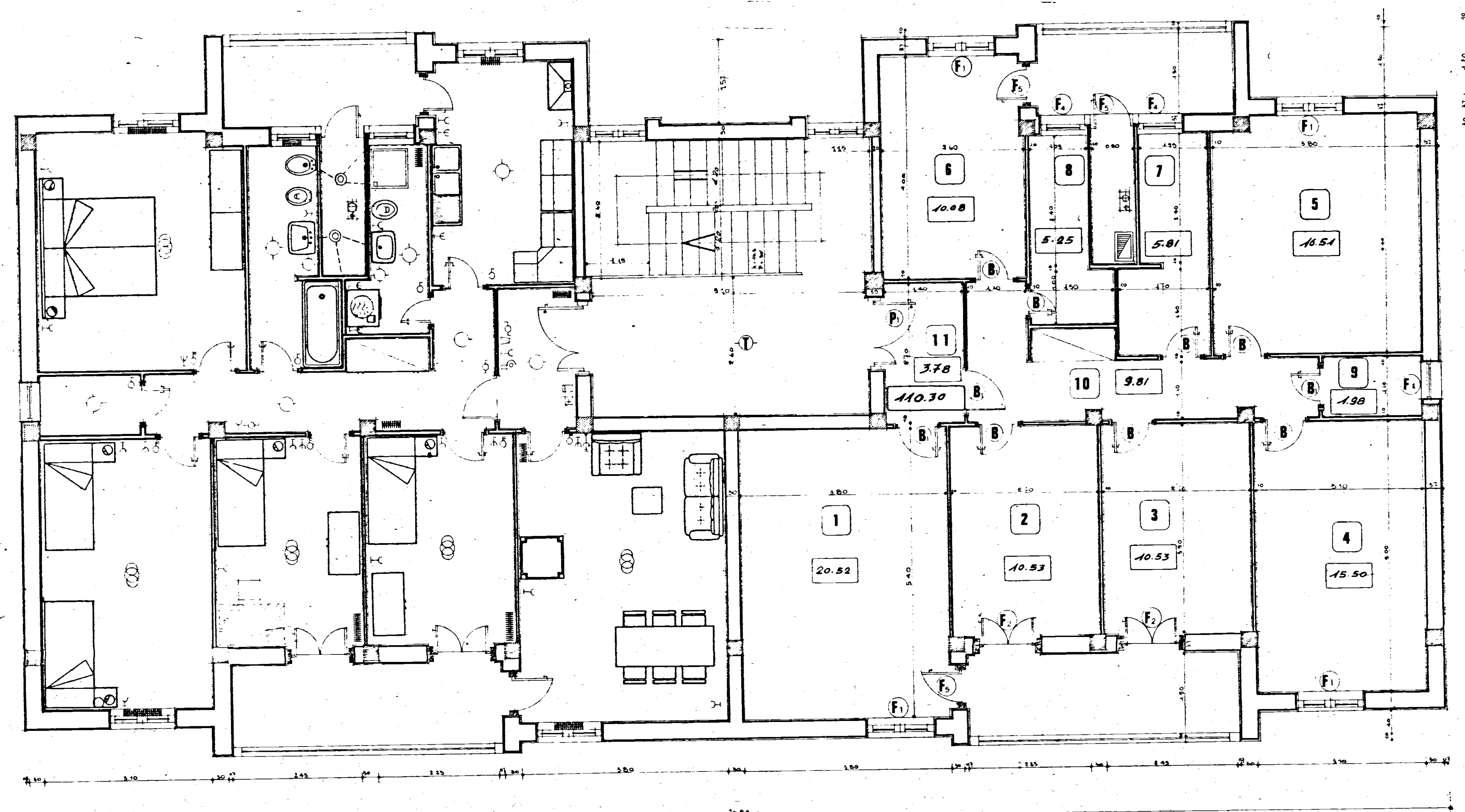
PIANTA TIPO
