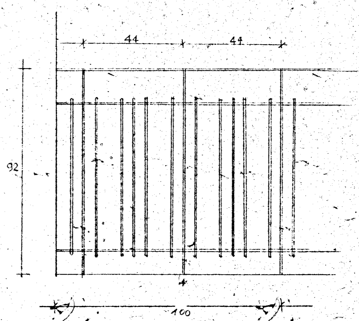
RINGHIERA ESISTENTE. RAPP. 1/10.
