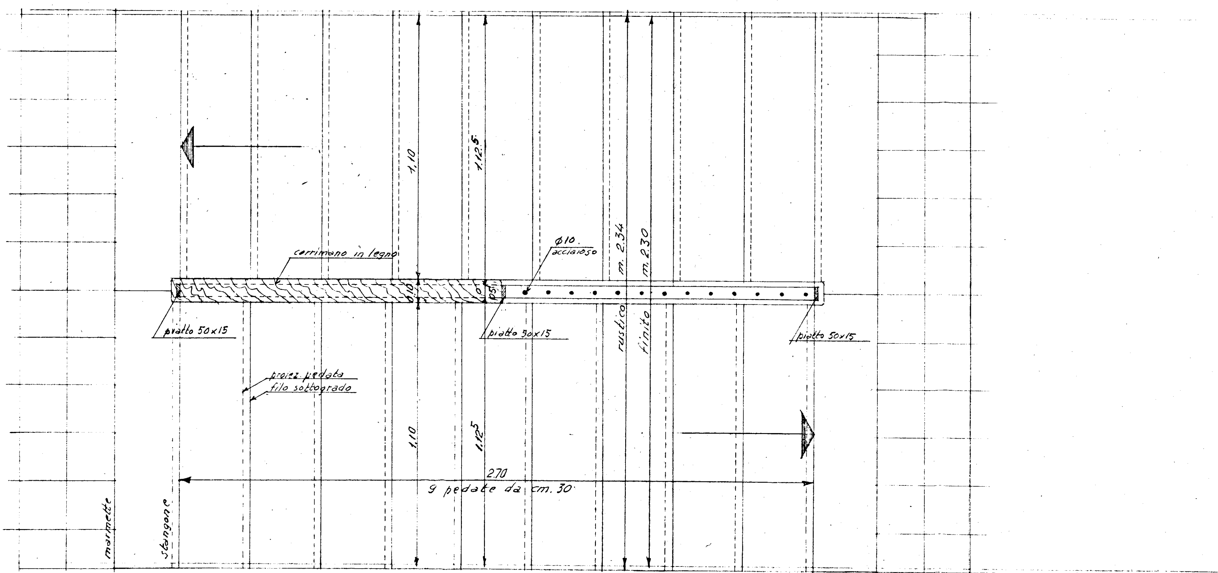
PIANTA - RAPP. 1:10
