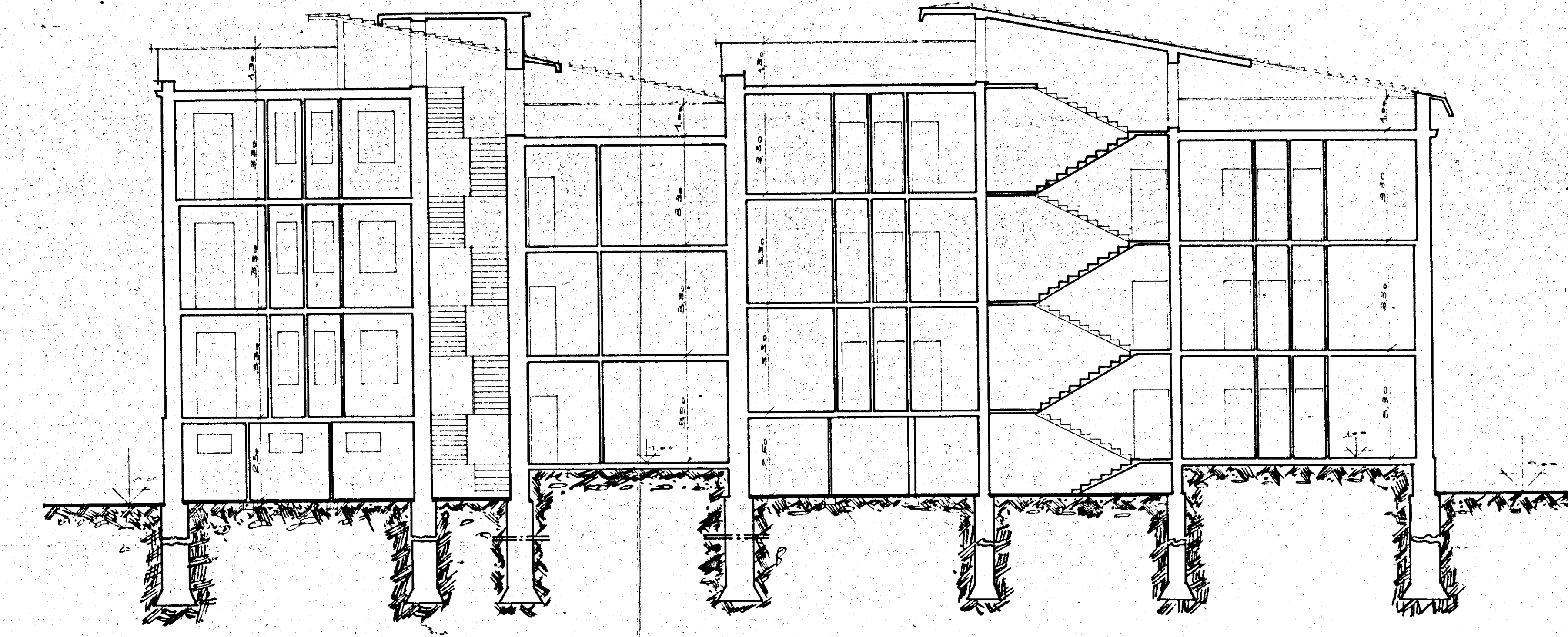
SEZIONE LONGITUDINALE
