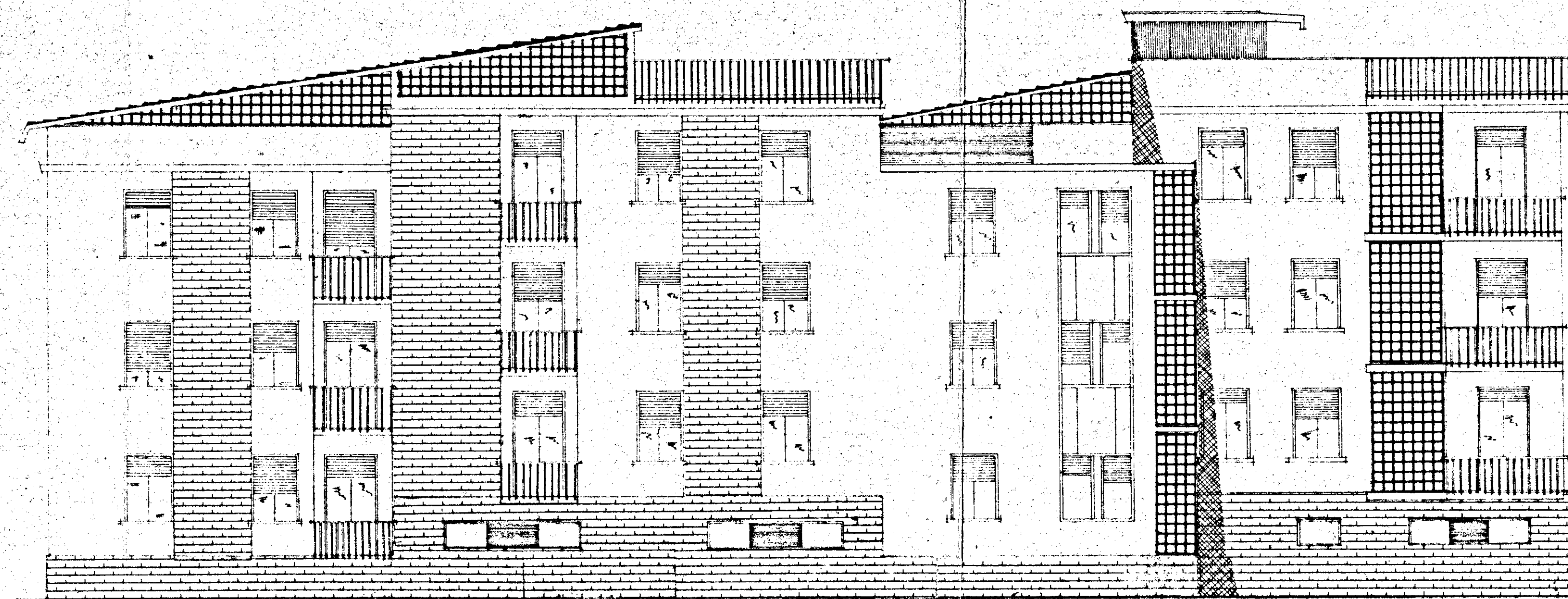
PROSPETTO POSTERIORE
