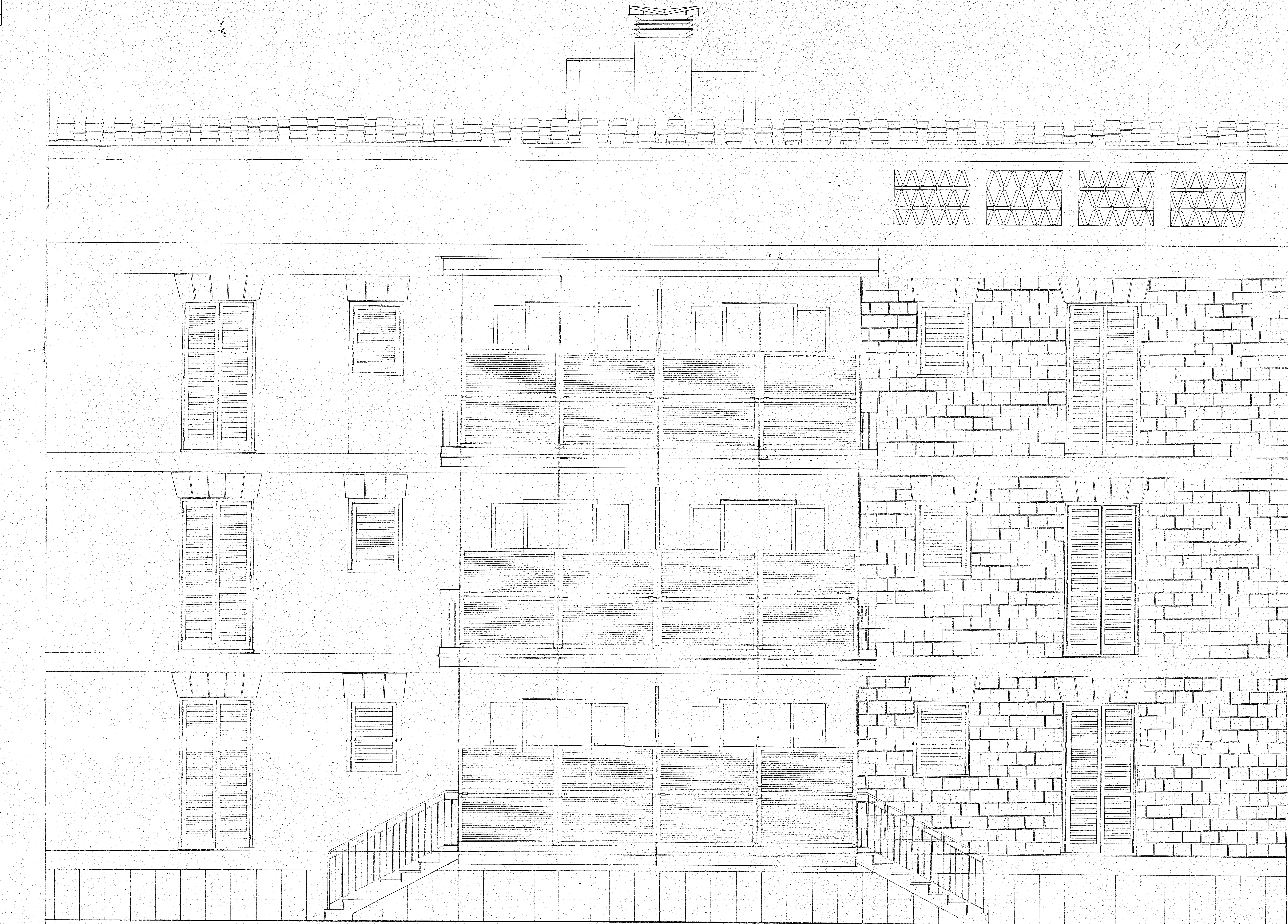
PROSPETTO
