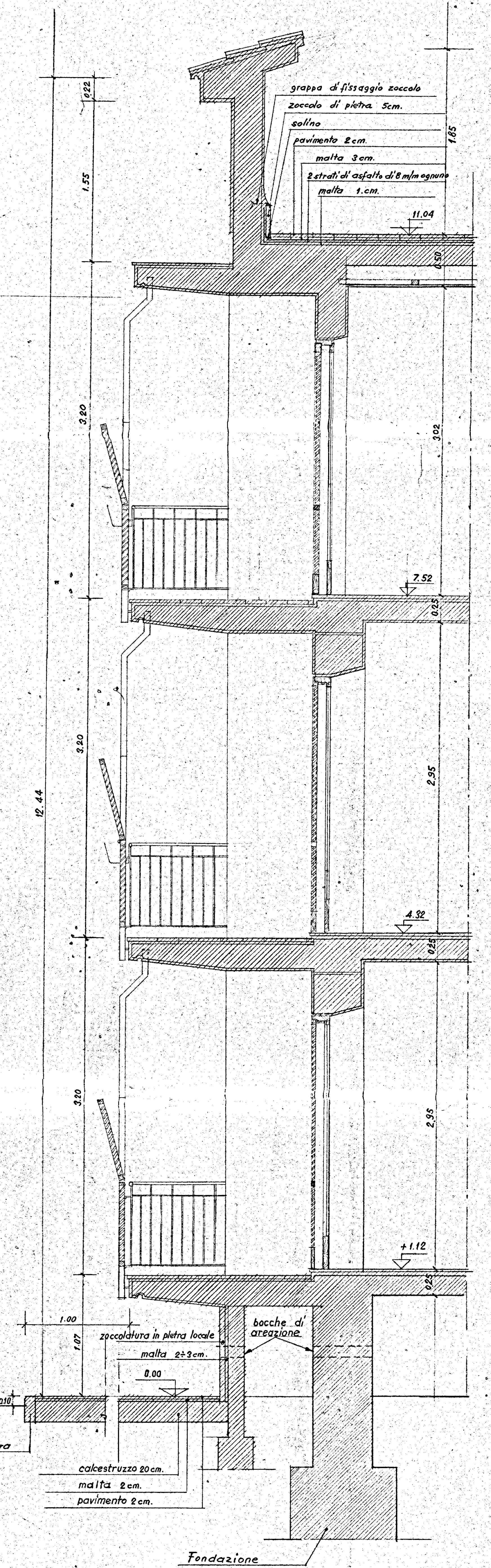
SEZIONE A-A
