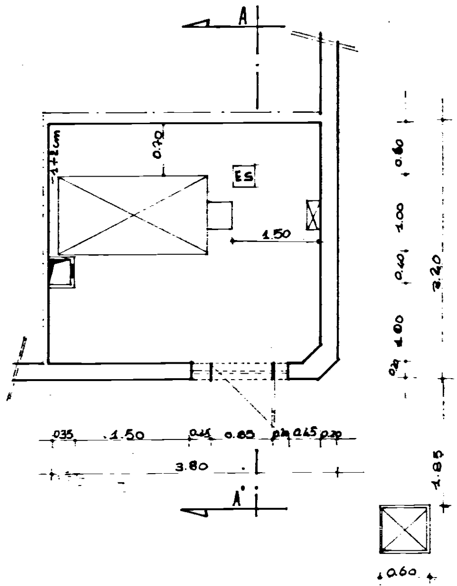
RILIEVO PIANTA CENTRALE TERMICA
