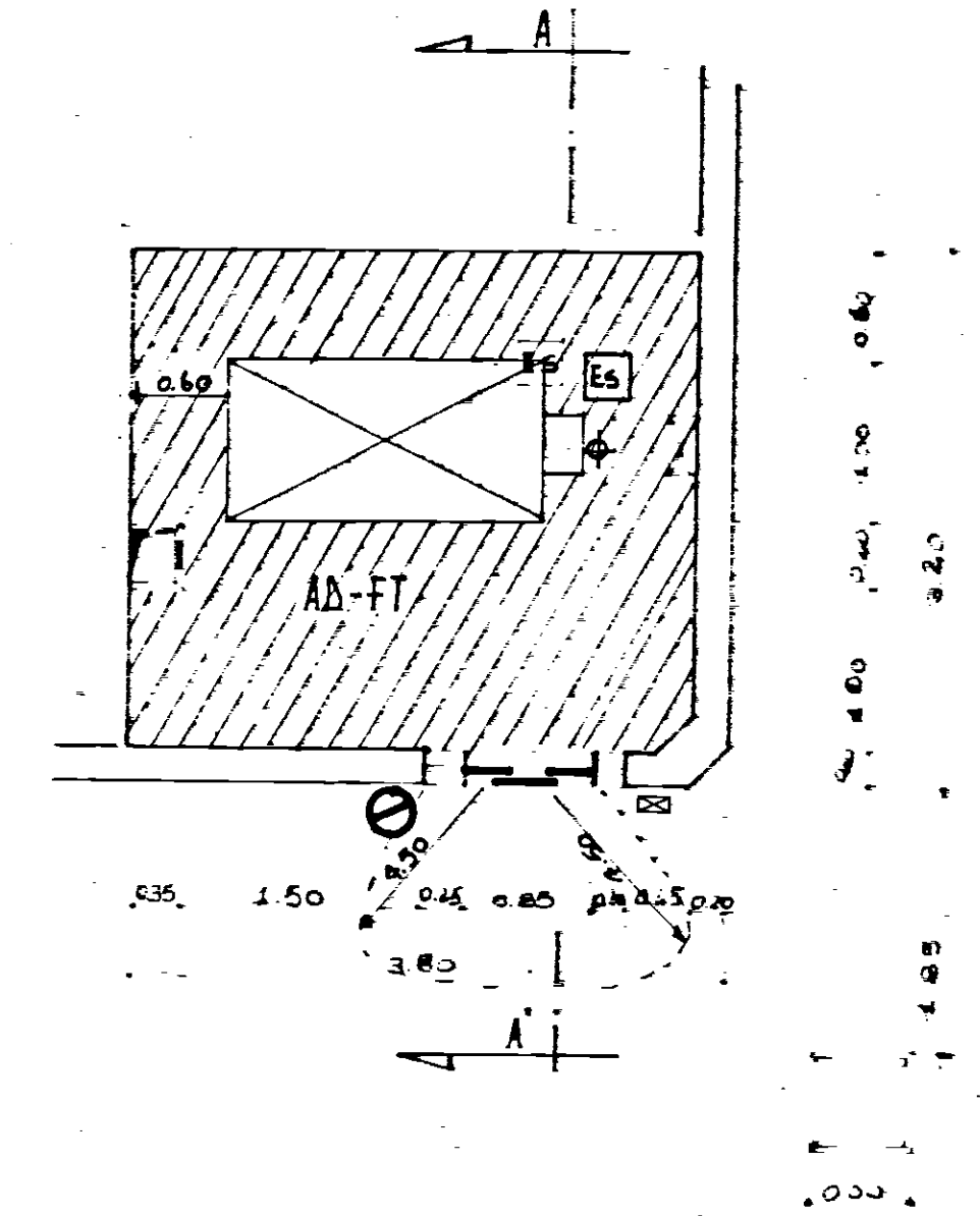
RILIEVO PIANTA CENTRALE TERMICA
