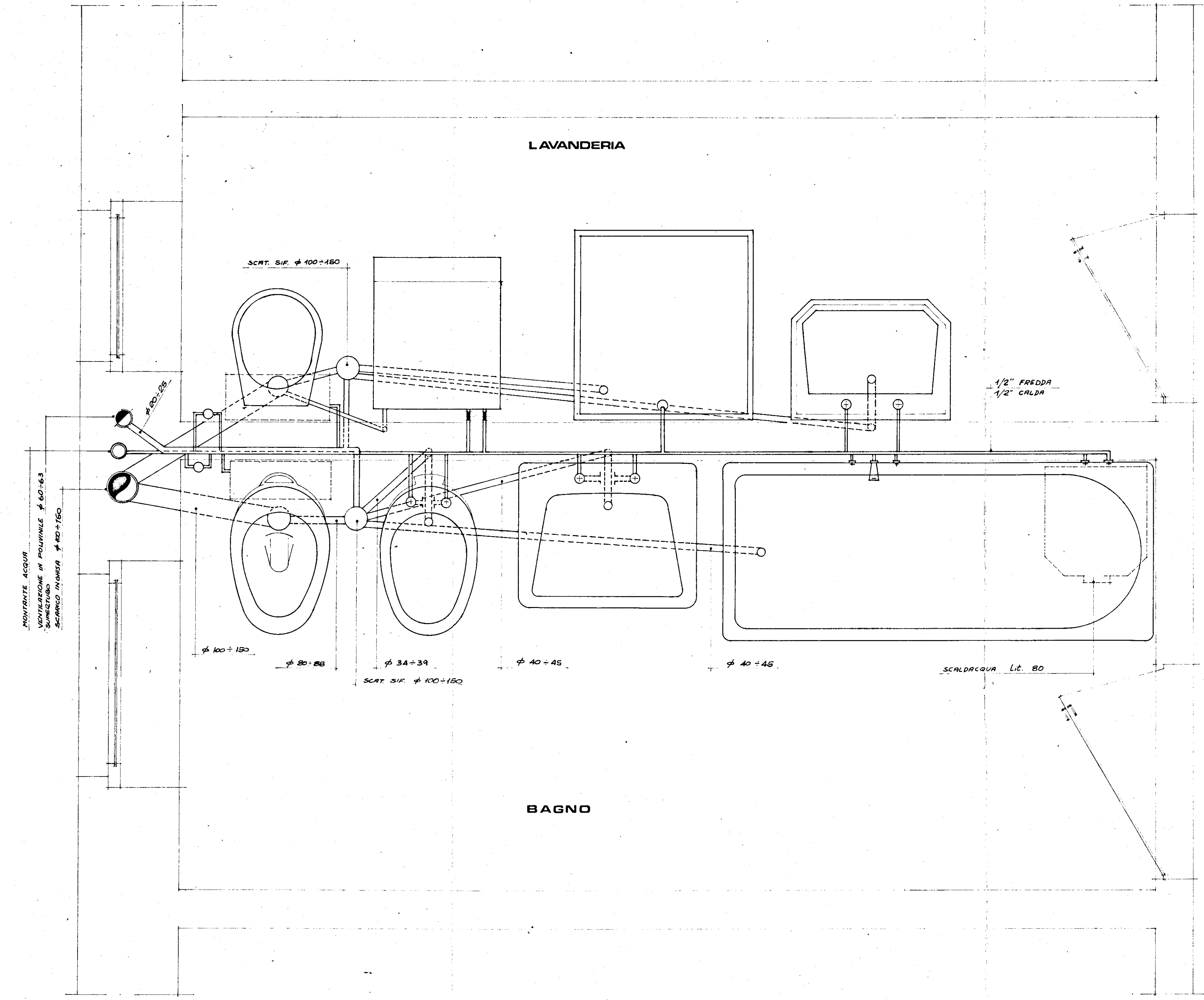
PIANTA r. 1:10
