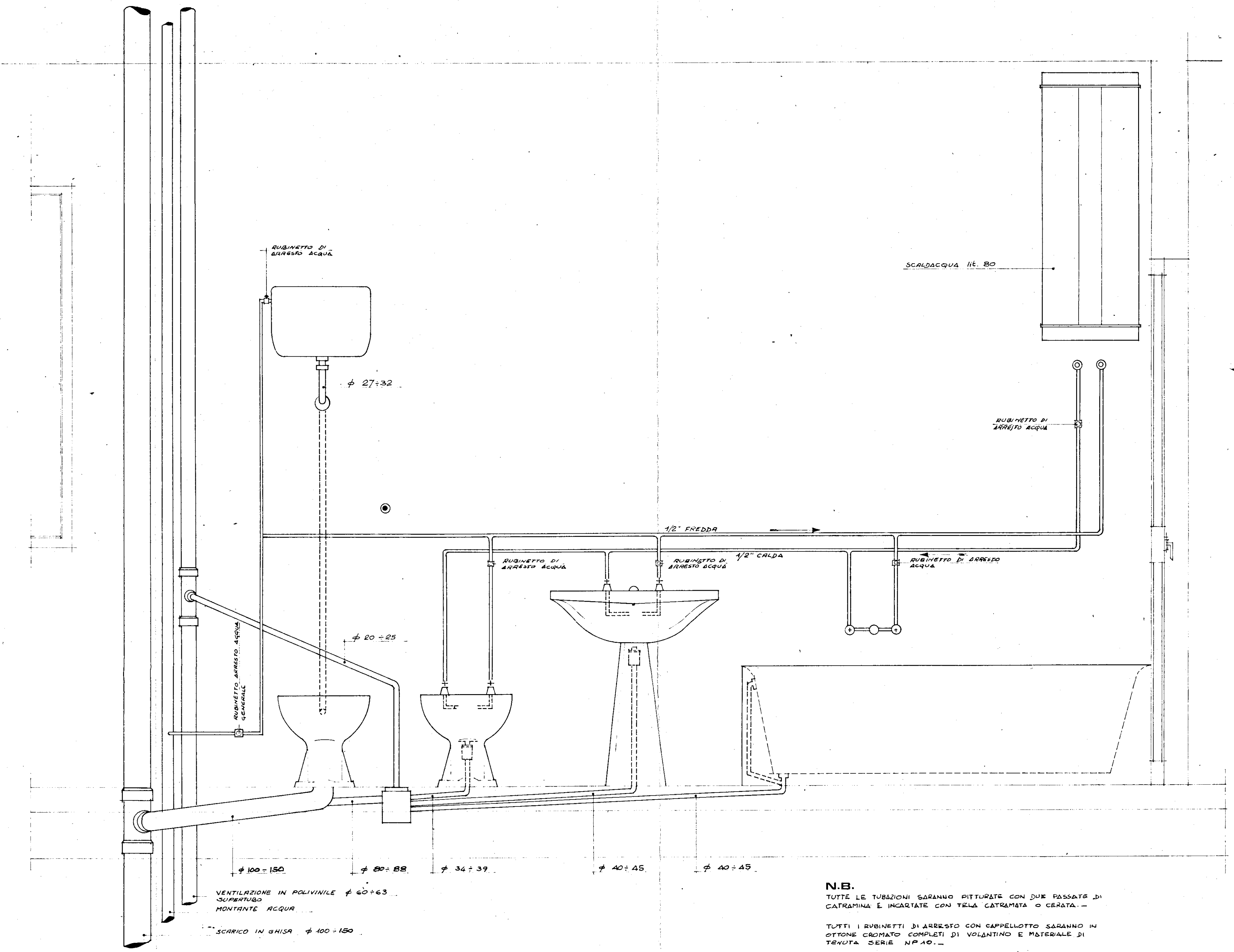
SEZIONE r. 1:10
