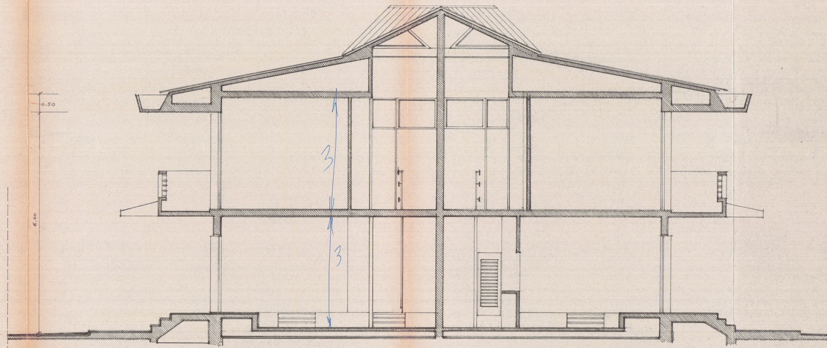
sezione sull'asse A-B
