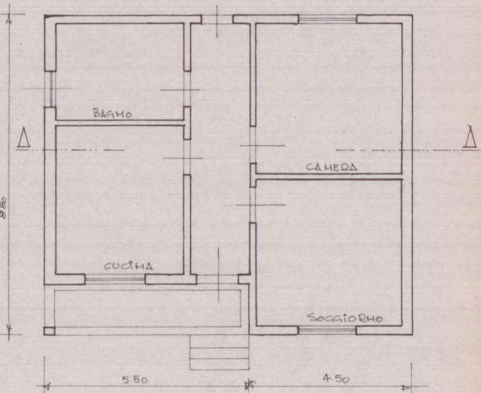
PIANTA P.T. ESISTENTE
