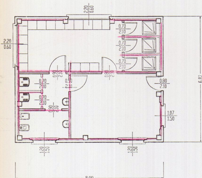
Pianta scala 1:100
