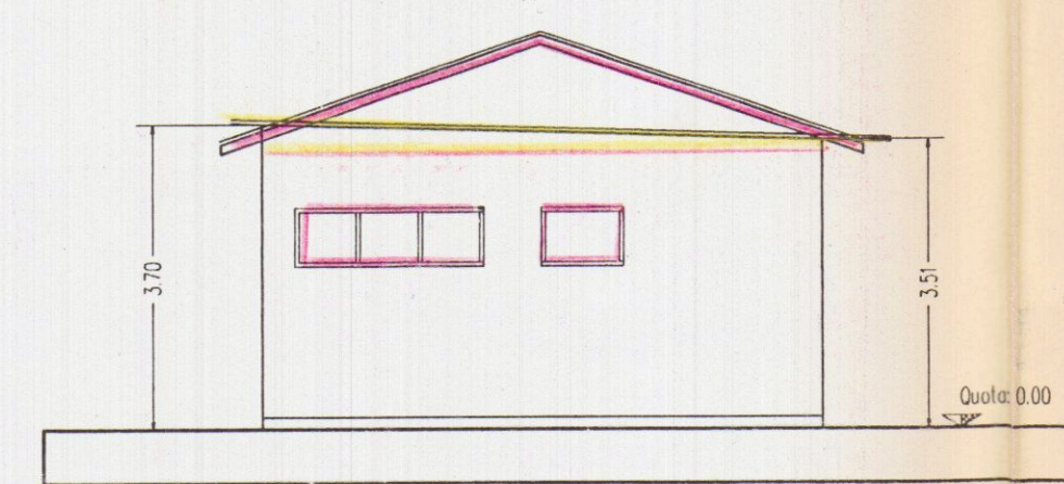
prospetto ovest
