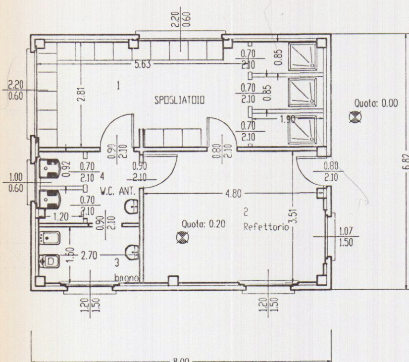
Pianta scala 1:100
