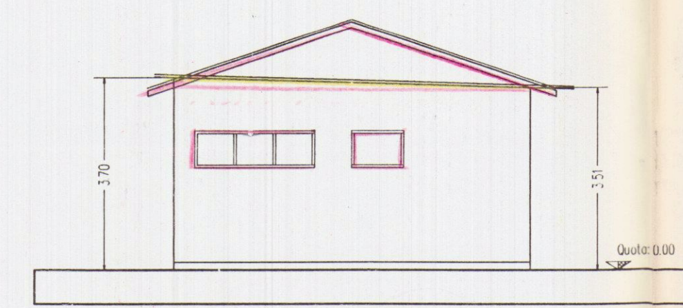
prospetto ovest
