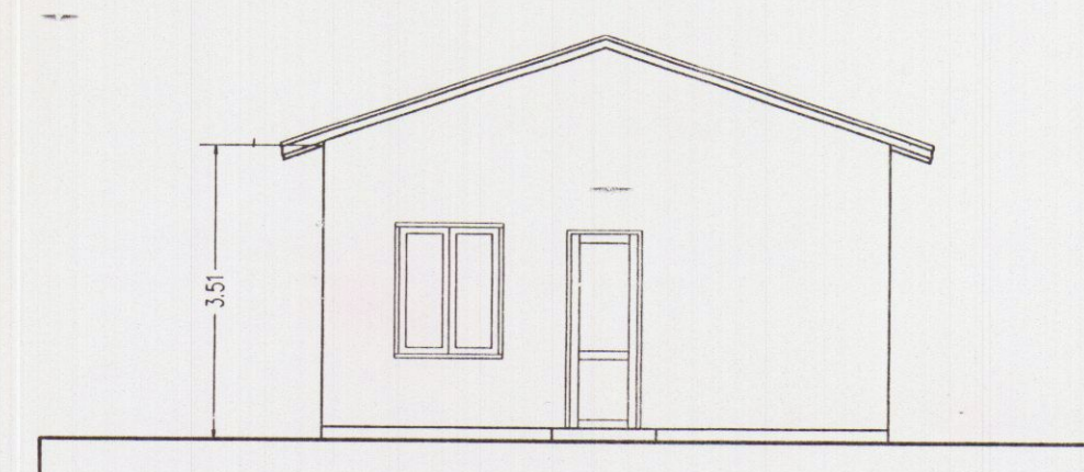
prospetto EST
