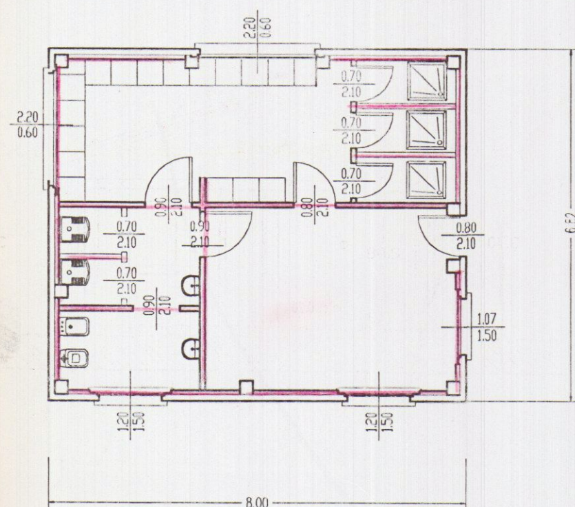
Pianta scala 1:100
