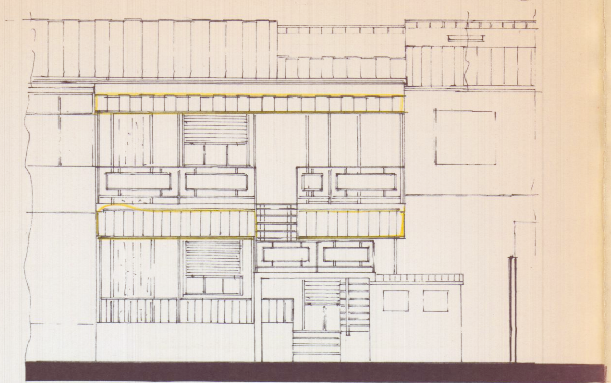
— PROSPETTO SUD attuale —
