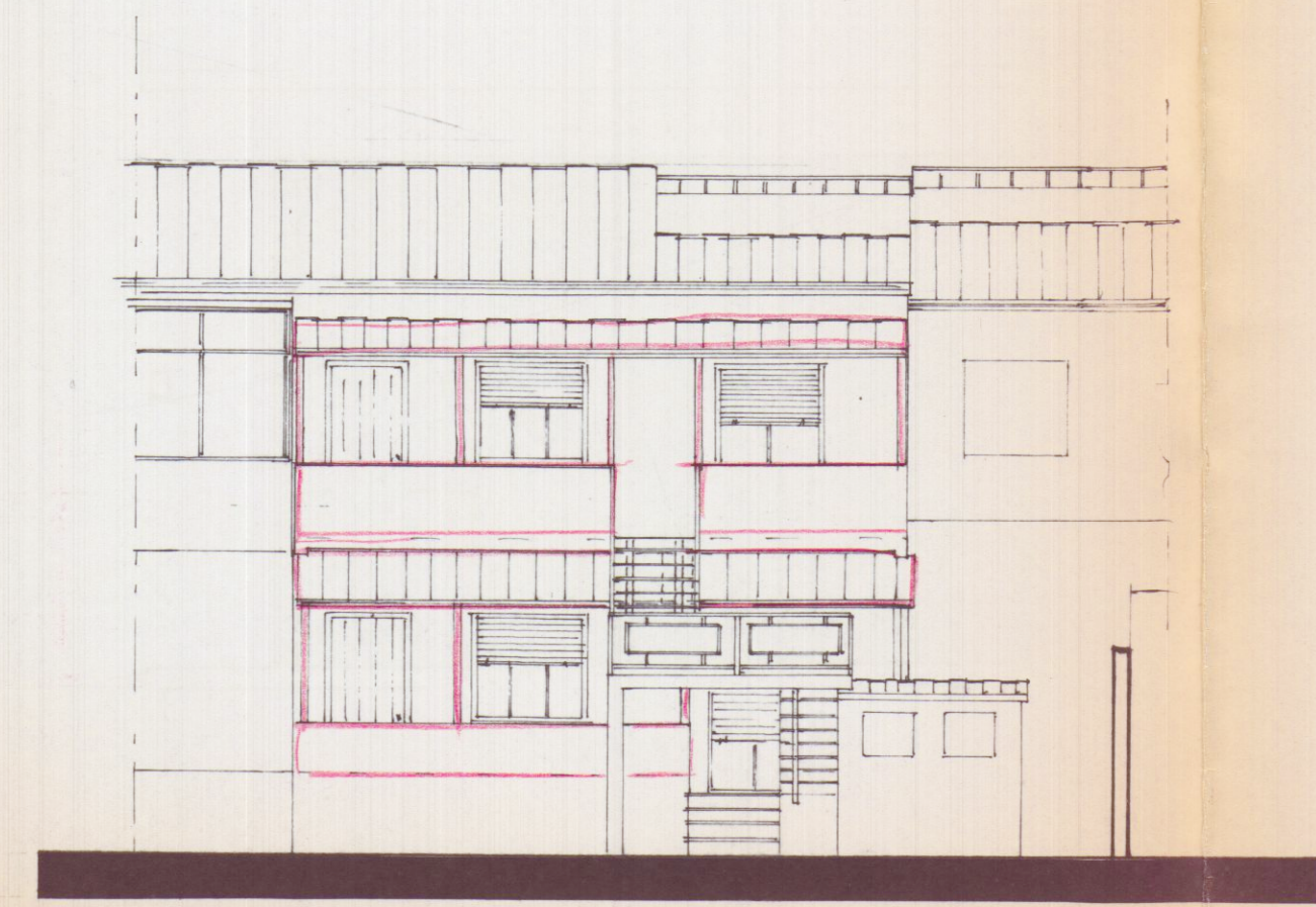
PROSPETTO SUD di progetto
