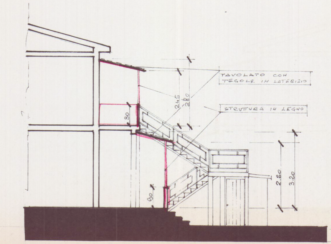
SEZIONE
