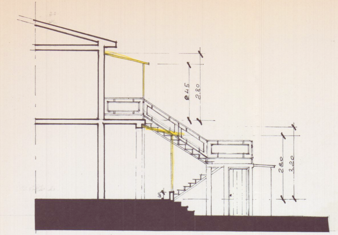
— SEZIONE —
