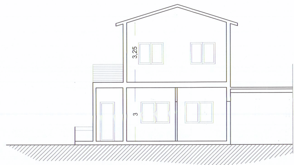
SEZIONE B-B
