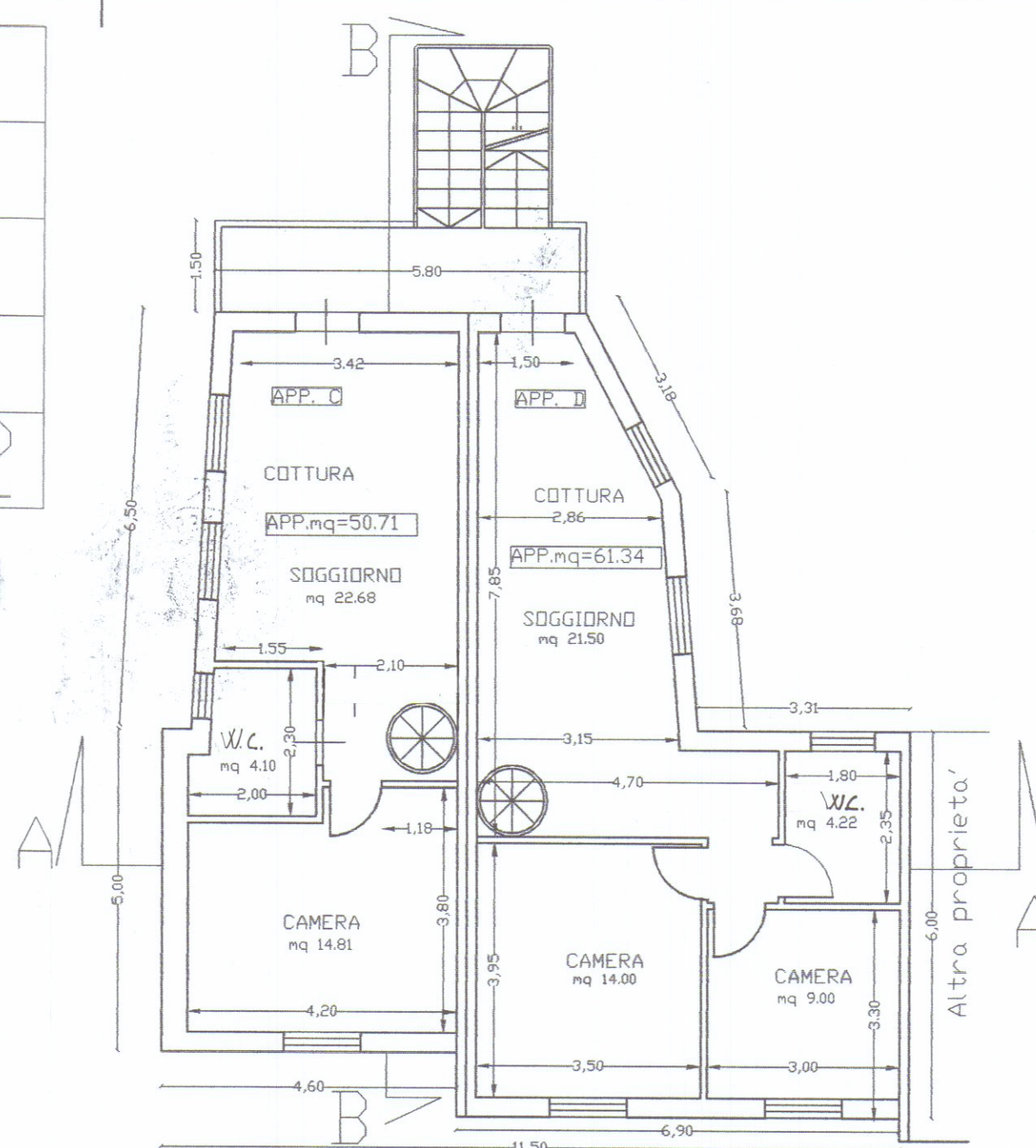
PIANO PRIMO
