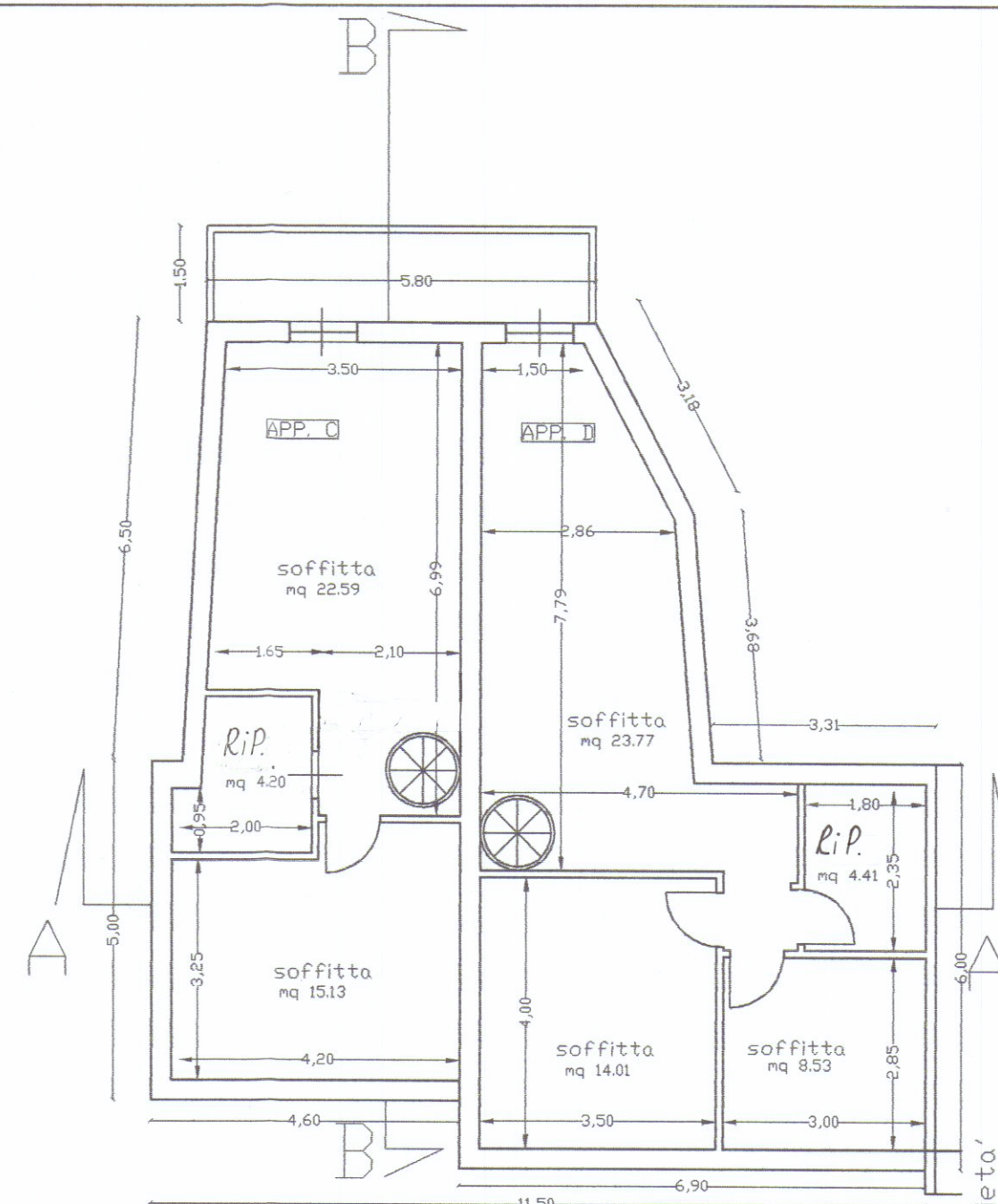
PIANO SOTTOTETTO
