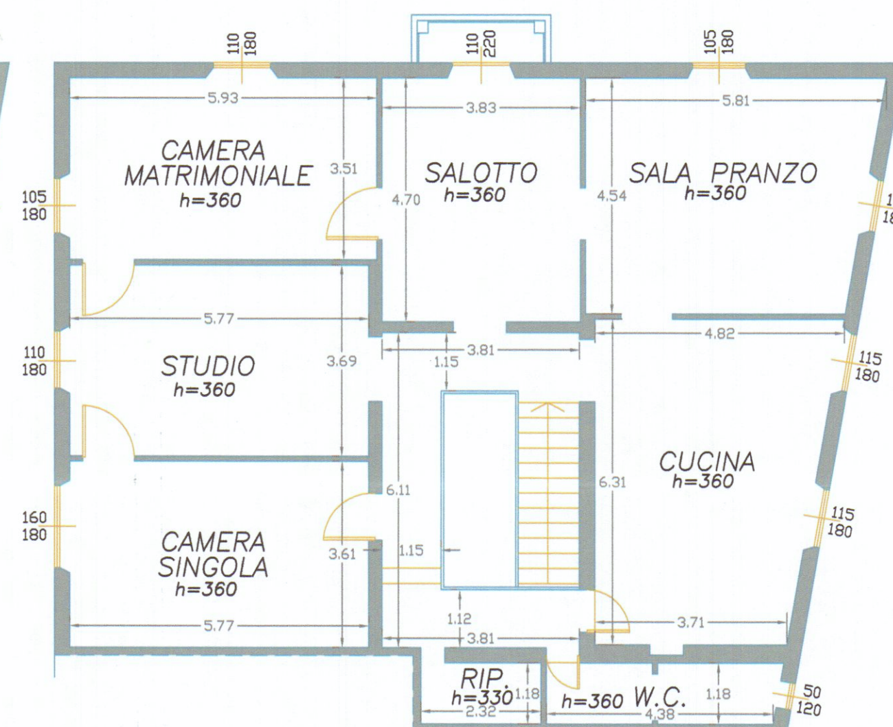
PIANO PRIMO Stato Attuale
