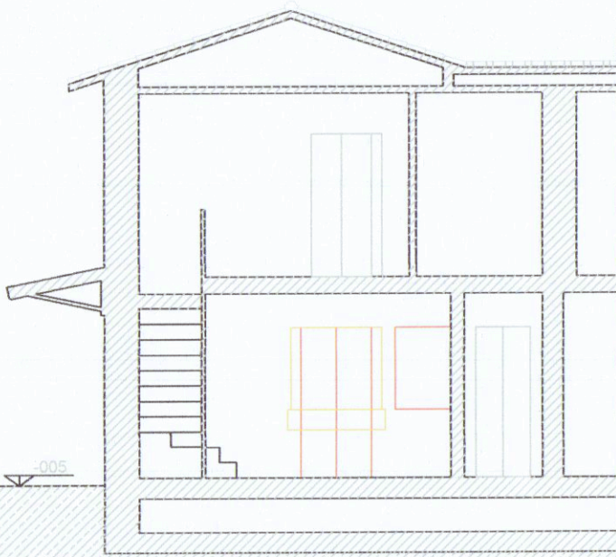
SEZIONE A-A' scala 1.100
