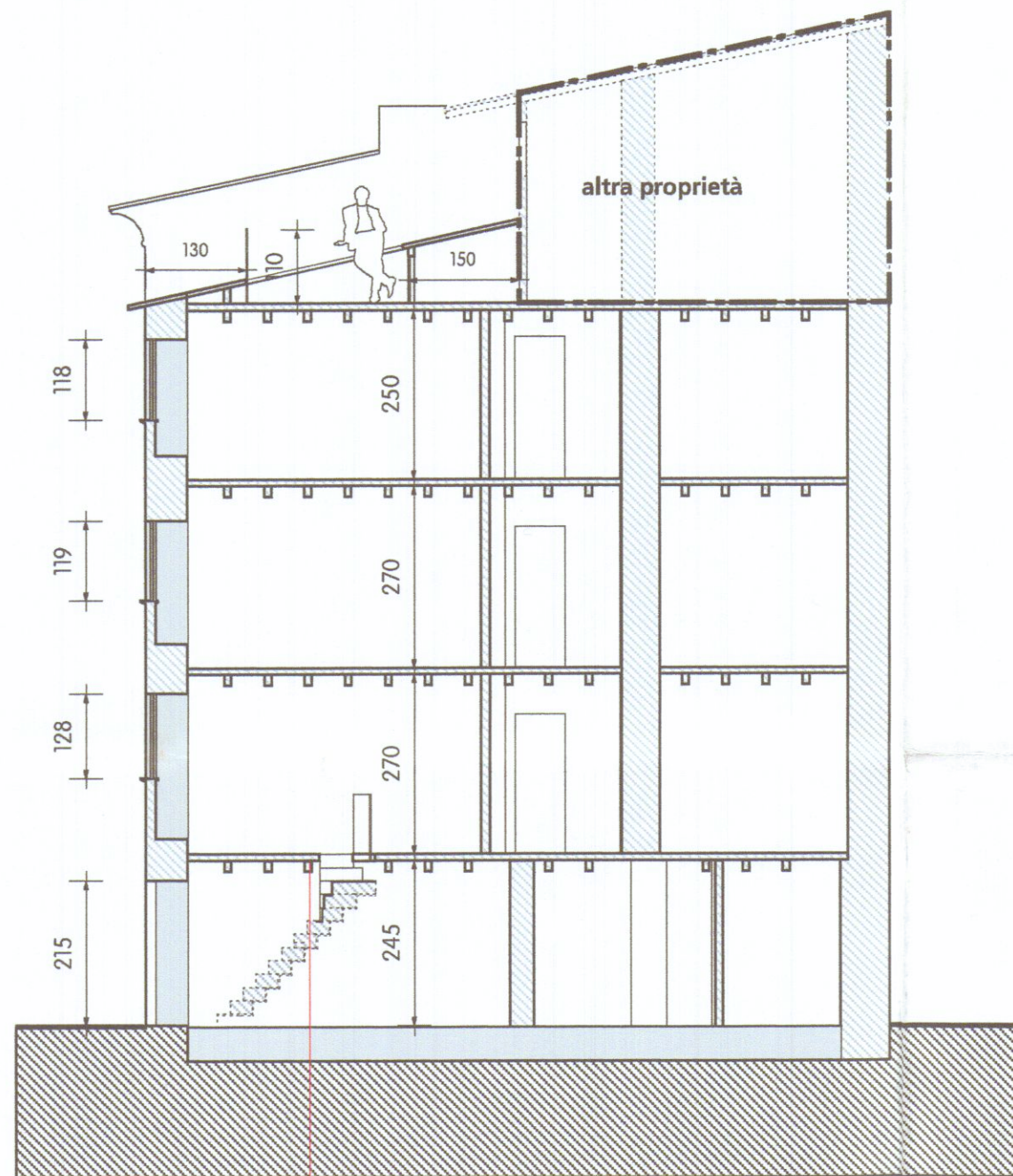
sezione scala 1: 100
