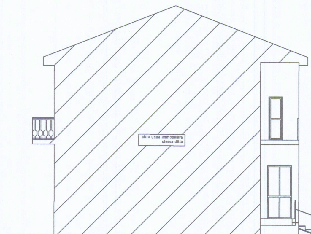
PROSPETTO EST
