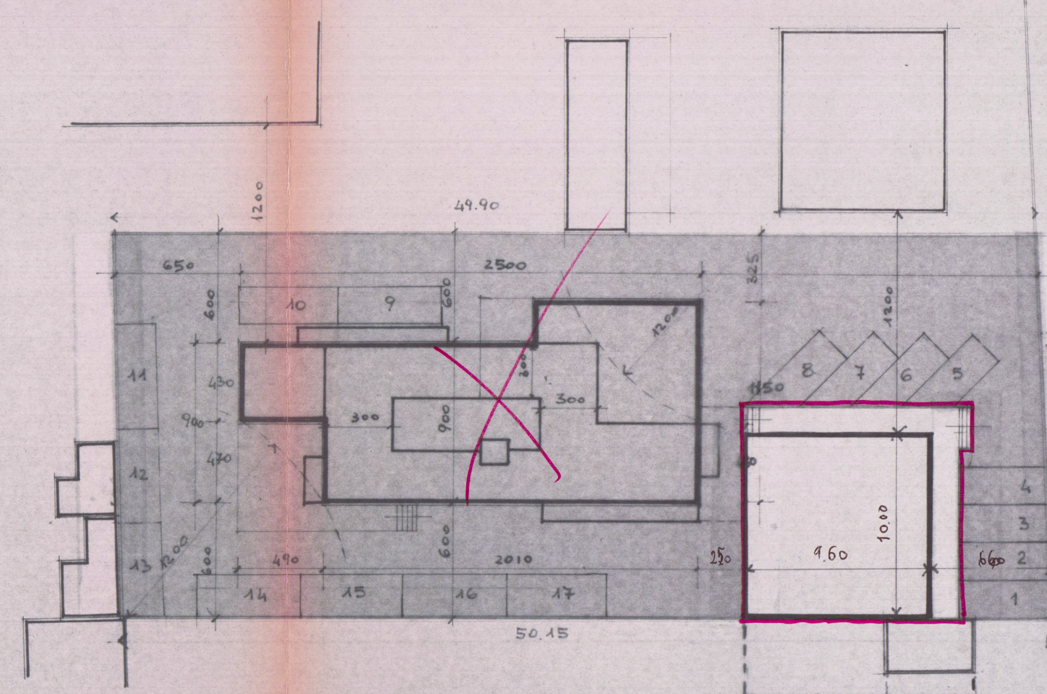
PLANIMETRIA RAPP. 1:200
