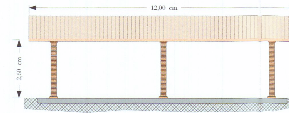
PROSPETTO EST E OVEST
