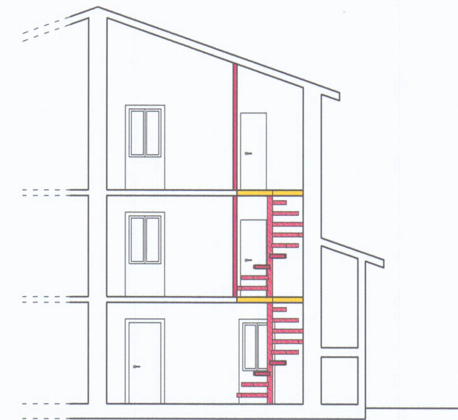
Sezione Y - Y 1
