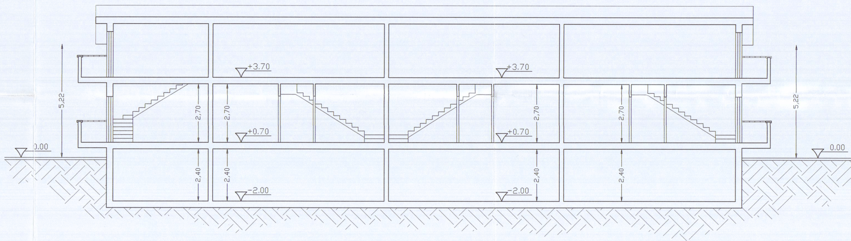
SEZIONE A-A
