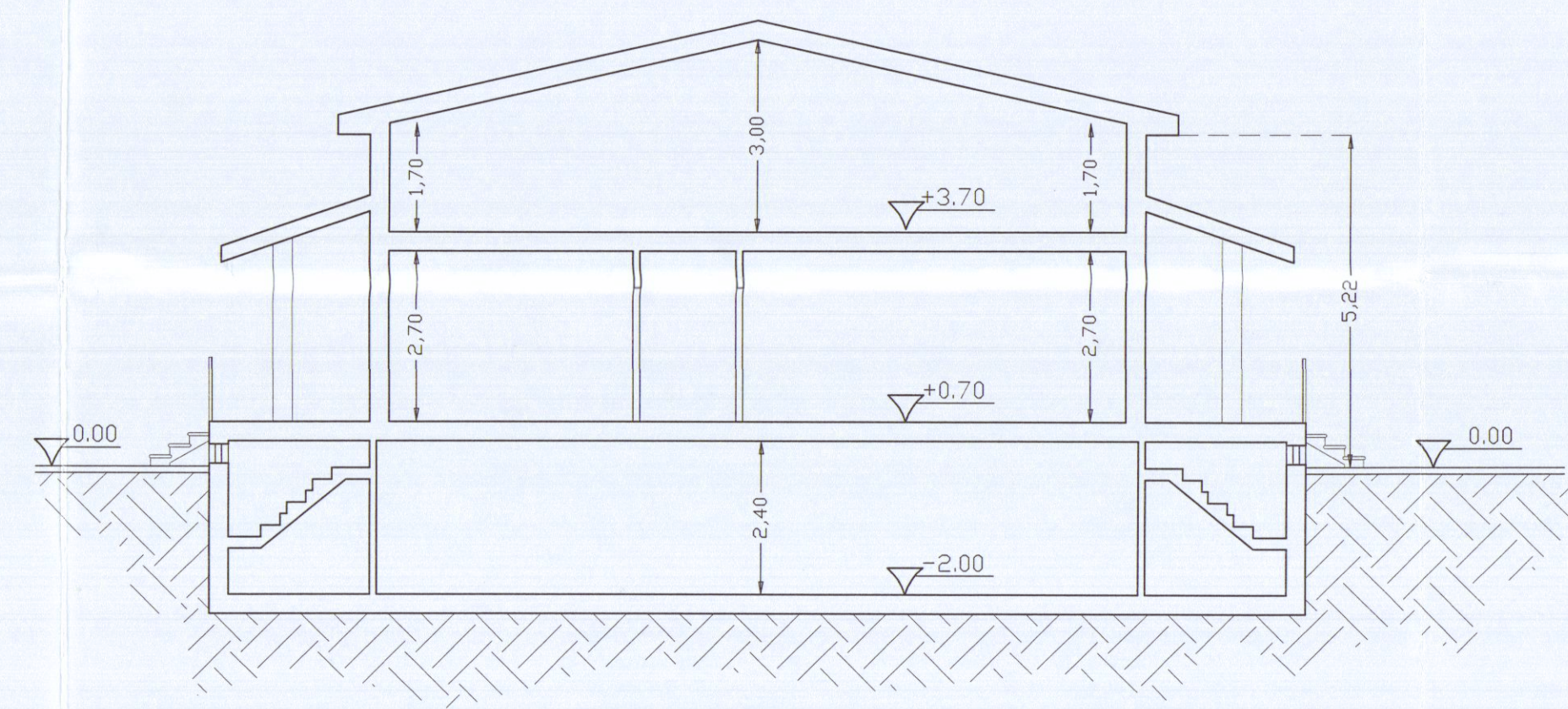
SEZIONE B-B
