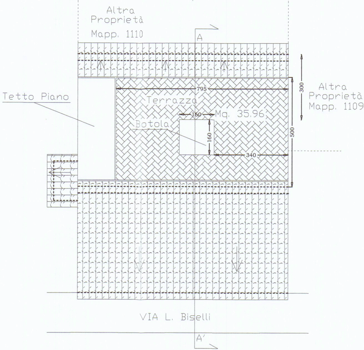
Pianta Copertura
