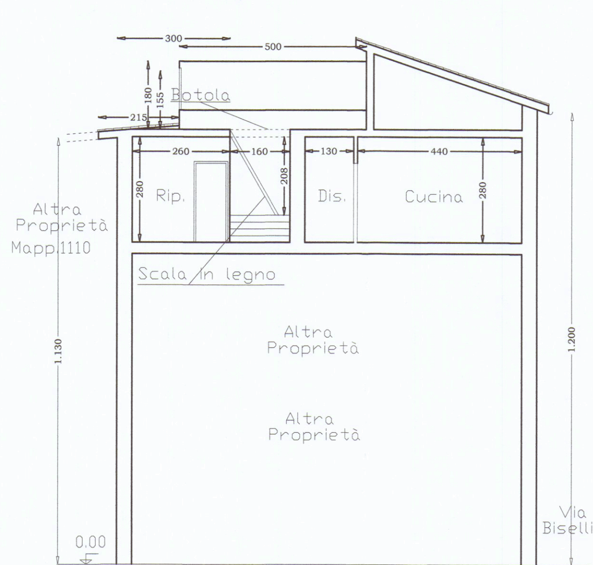
Sezione A-A'
