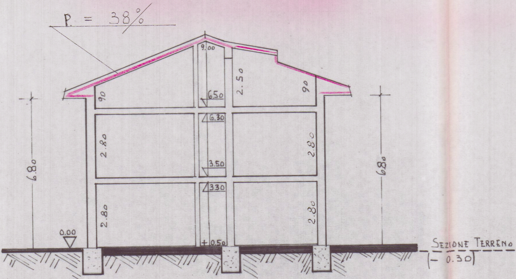
SEZIONE X-X
