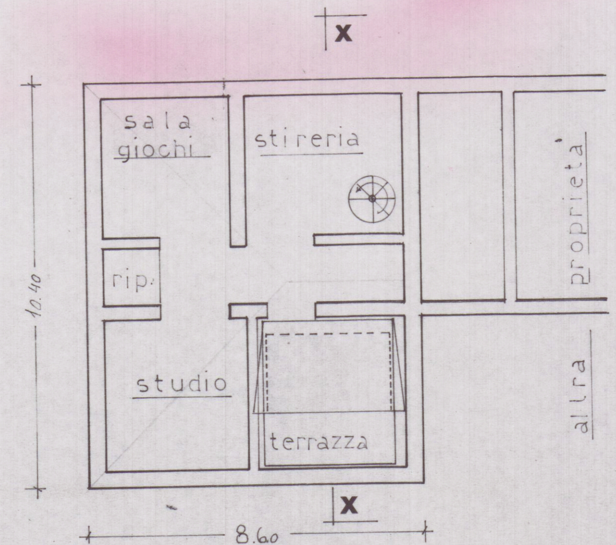
PIANTA SOTTOTETTO
