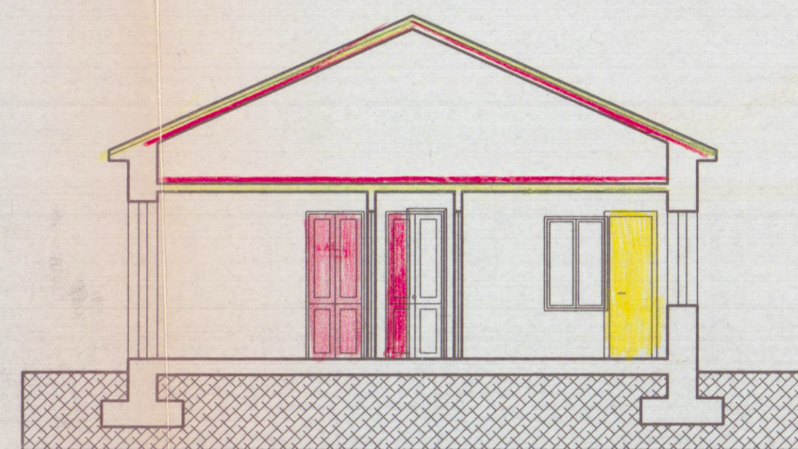
SEZIONE A-A
