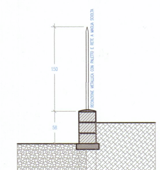
Sezione Tipo Muro in Bozzetti di cls
