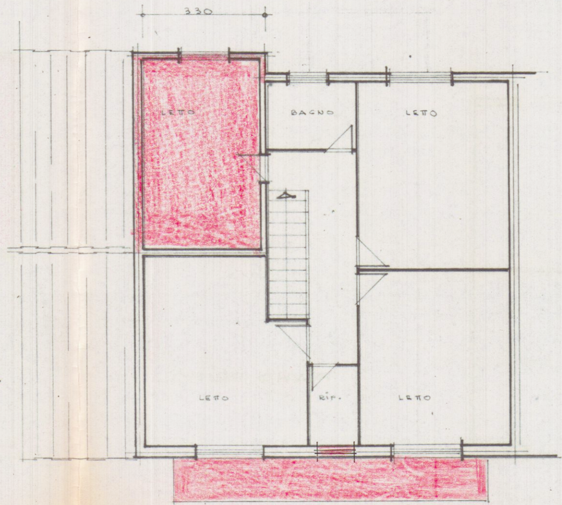
PIANO PRIMO
