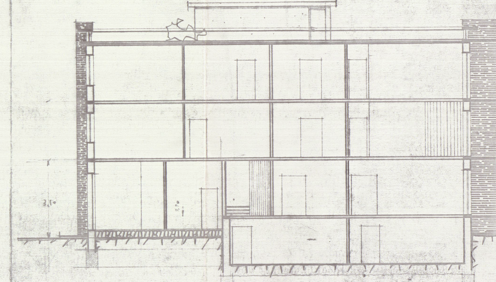
SEZIONE A-A
