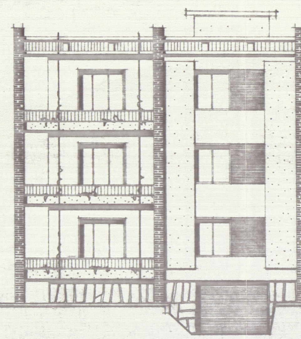
PROSPETTO SUD
