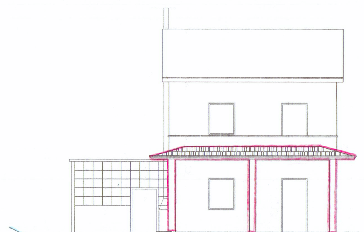
PROSPETTO SUD
