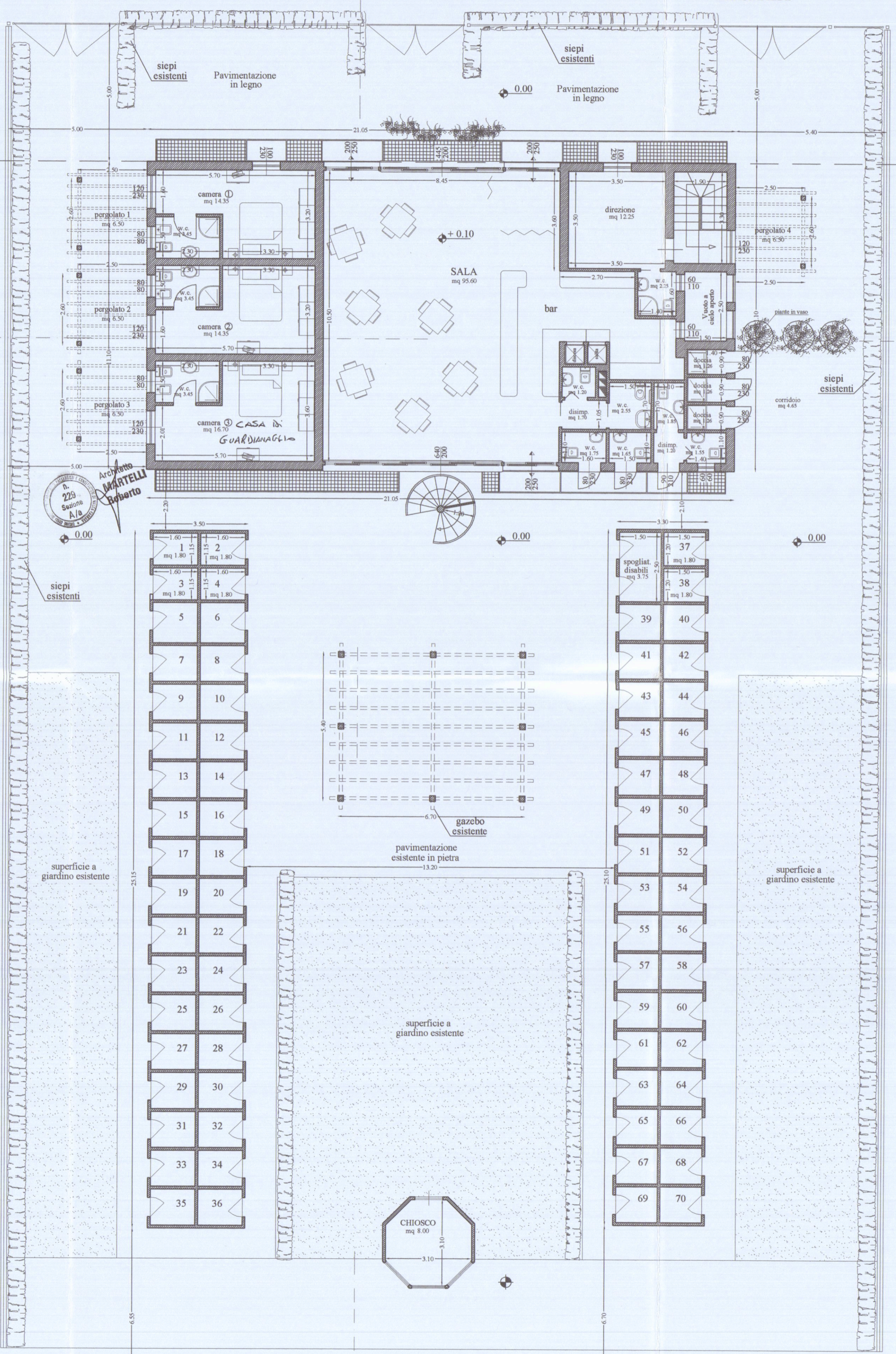
PIANTA PIANO TERRA
