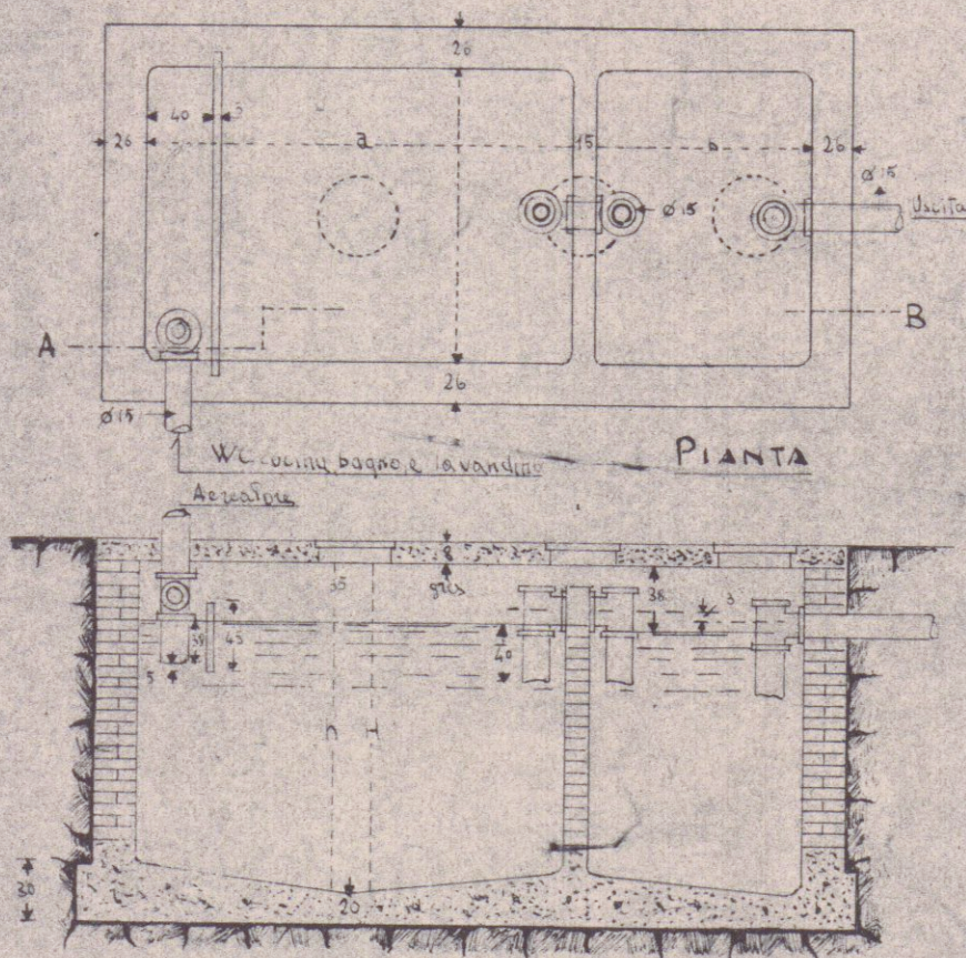
SEZIONE A-B
