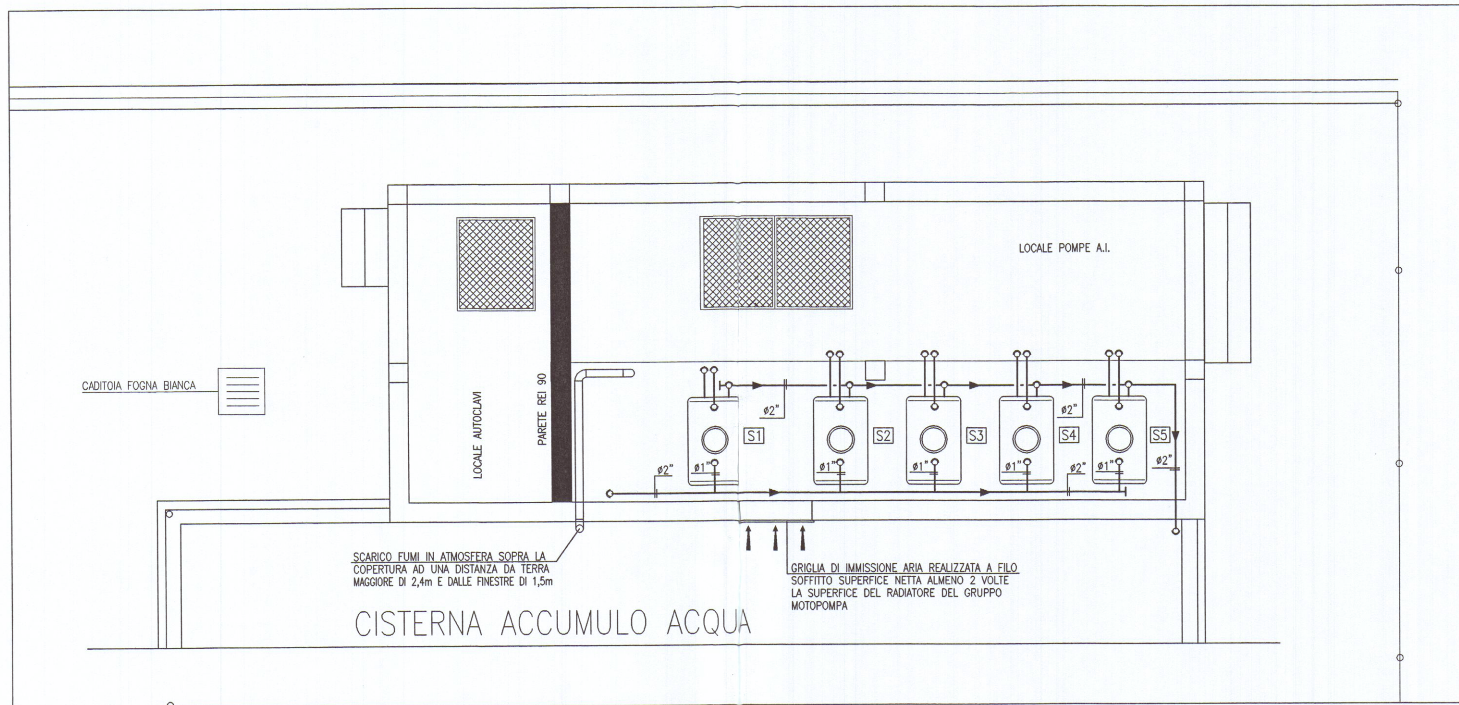
PIANTA PIANO AMMEZZATO
