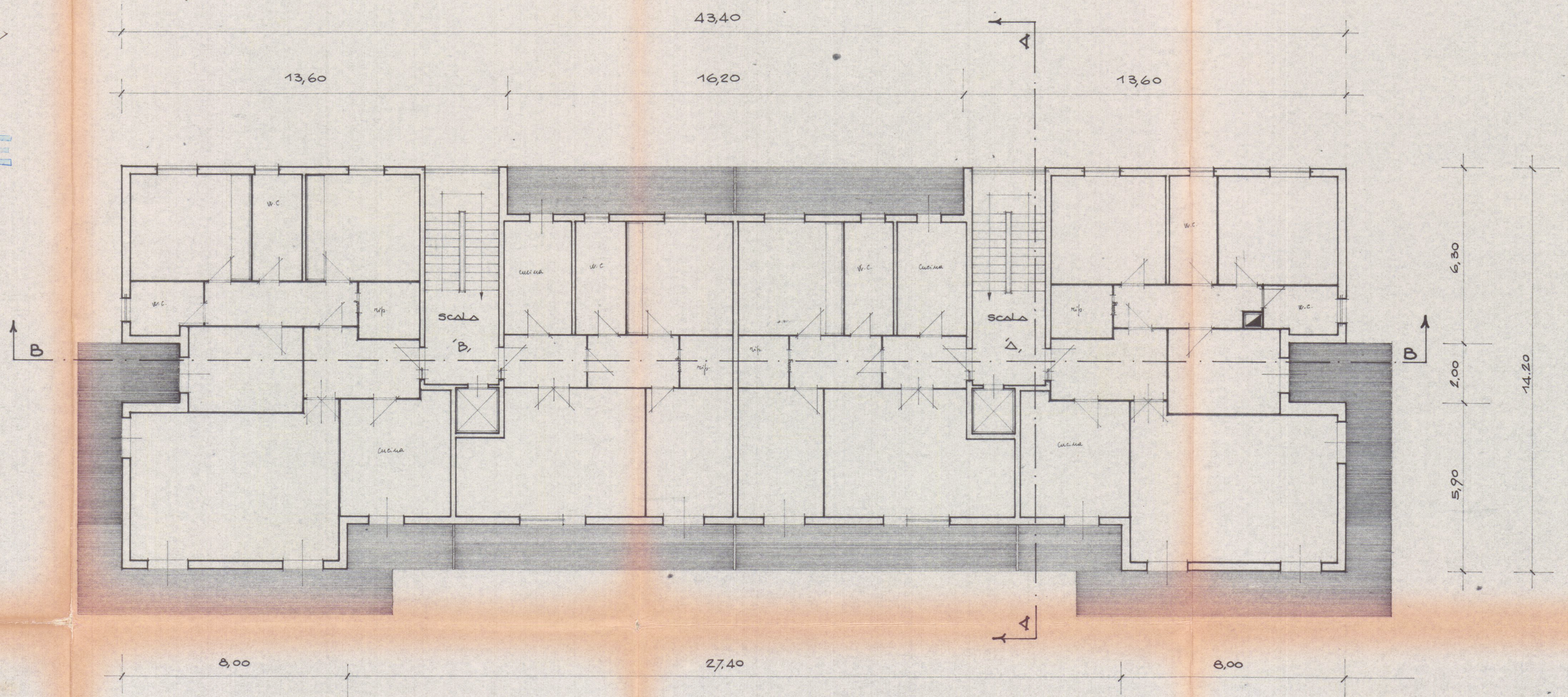
PIANTA PIANO 4° E 5°
