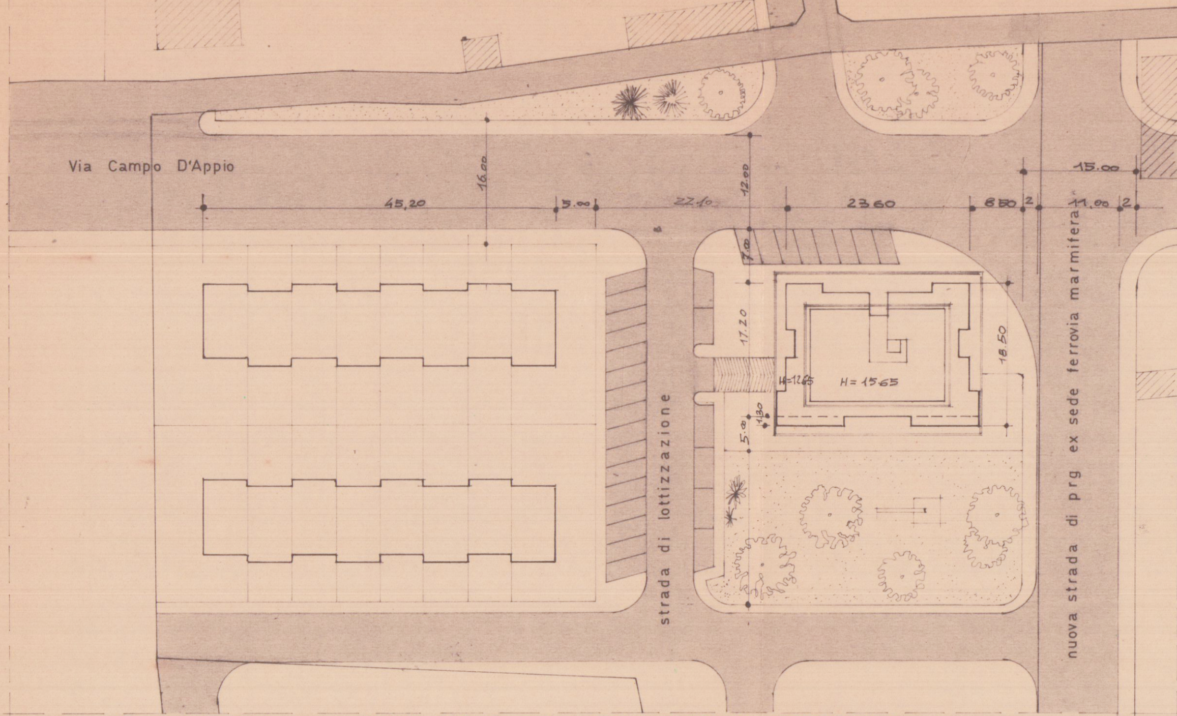
PLANIMETRIA scala 1:500 COME DA LOTTIZZAZIONE APPROVATA
